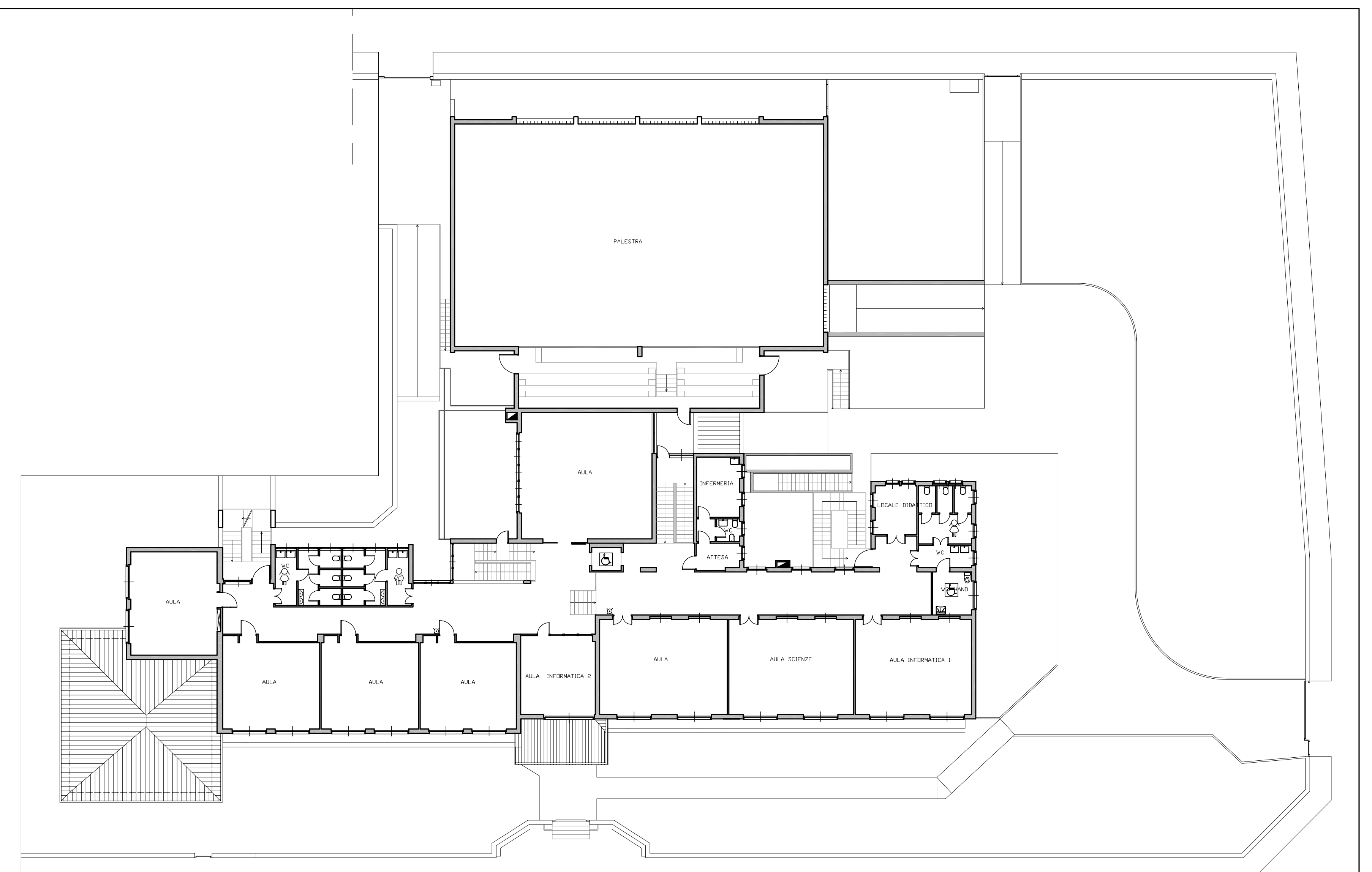
SCUOLA ELEMENTARE ADA NEGRI PIANO PRIMO
