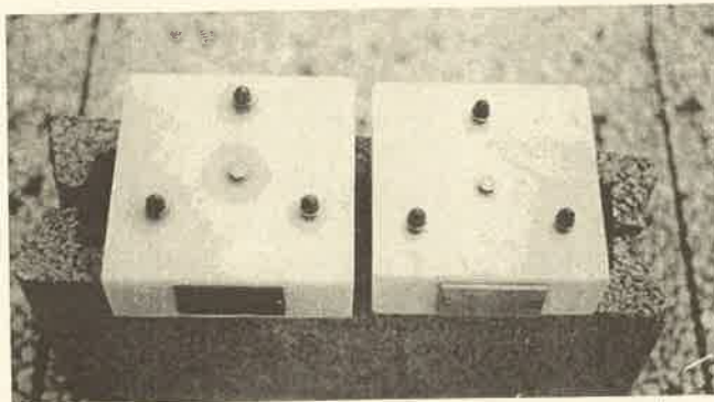
I blocchetti di marmo utilizzati per gli studi sulla corrosione
