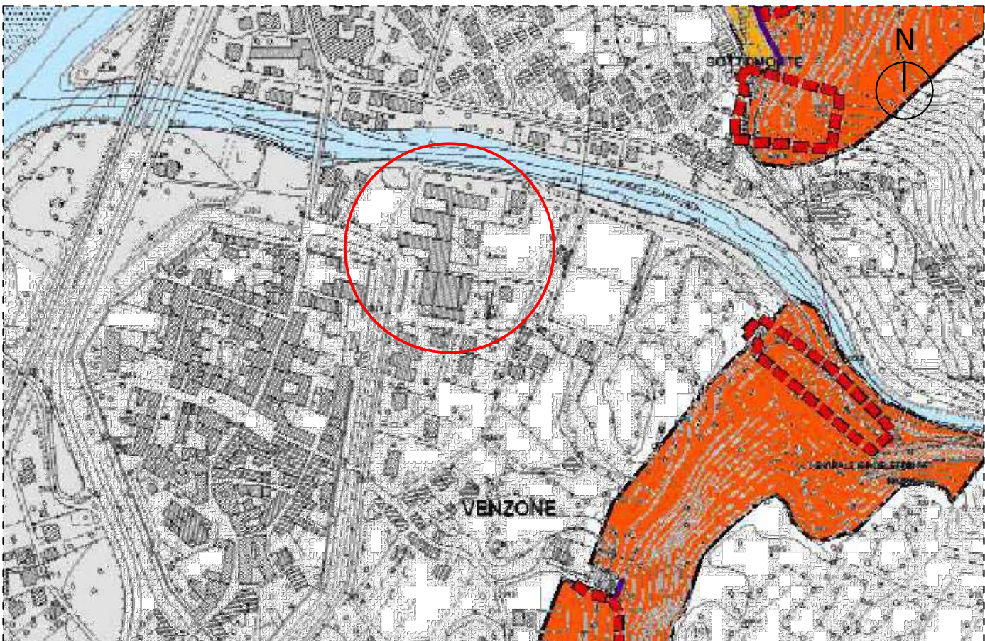
Estratto carta della pericolosità geologica / scala 1:5000
