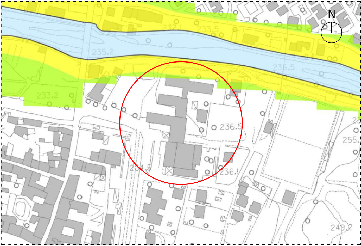
Estratto carta della pericolosità geologica / scala 1:5000
