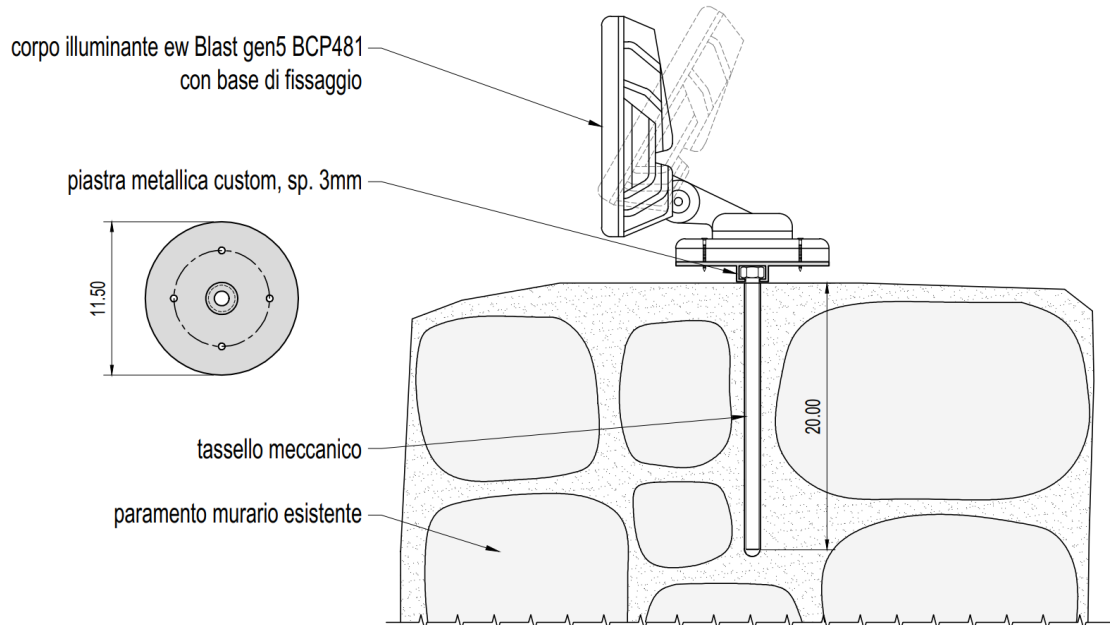
Figure 41: Progetto – Dettaglio ancoraggio corpi illuminanti su paramento orizzontale
