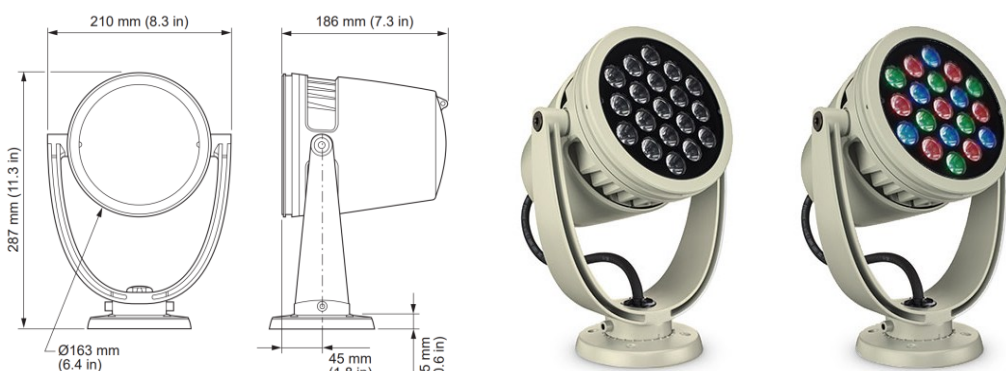
Figure 55: Progetto: ew Burst BCP463 G3 con luce bianca 3000K e Color Burst Intellihue BCP462 G3 con luce RGBMW
