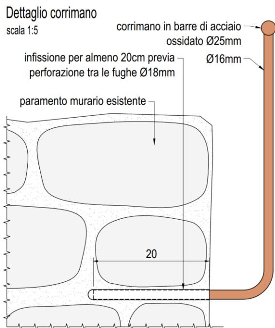
Figura 15: Progetto – Dettaglio corrimano in acciaio ossidato
