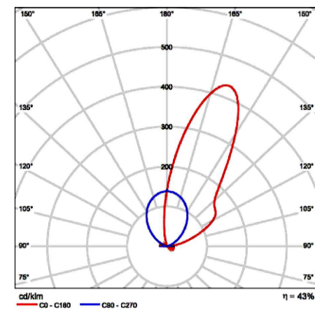
Fotometria tipo ottica LED Wall Washer 3000k
