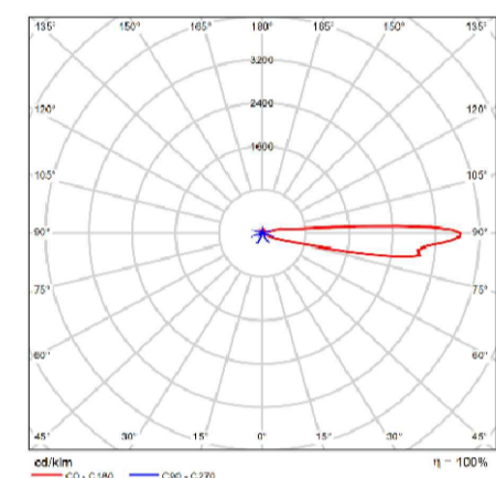
Fotometria tipo segnappasso LED 3000k
