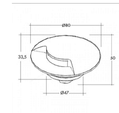
Tipico apparecchio segnappasso ad incasso a pavimento/terreno per sorgenti LED, IP68
