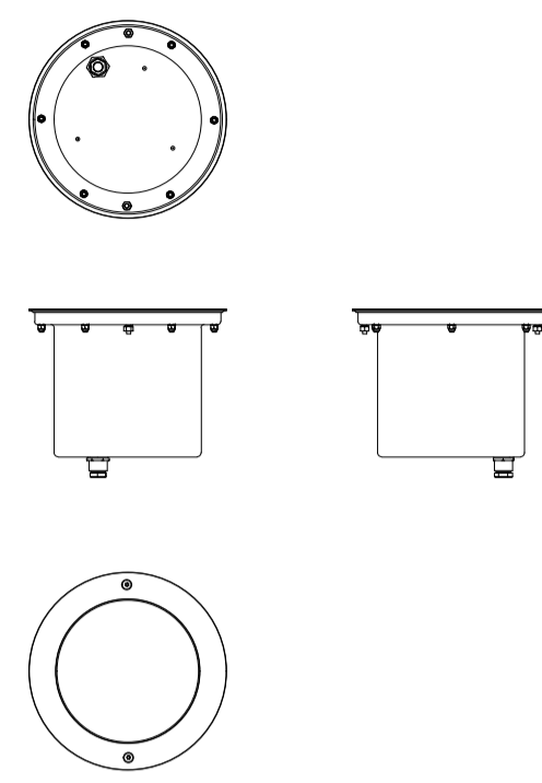
Tipico apparecchio ad incasso a pavimento/terreno per sorgenti LED, corpo e controcausa, IP68
