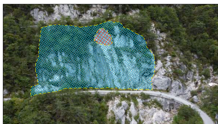
POSA GEOCOMPOSITO METALLICO TIPO STEELGRID HR50 O EQUIVALENTE 2.860,00 mq
