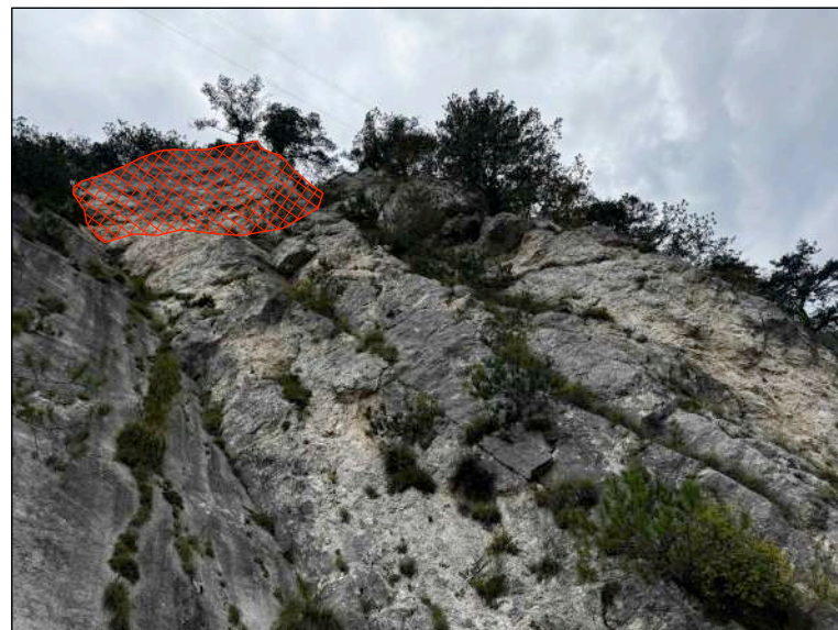
POSA PANNELLI DI RETE IN FUNE TIPO MACCAFERRI HEA PANELS O SIMILARE n°6 - 6 x 3 m
