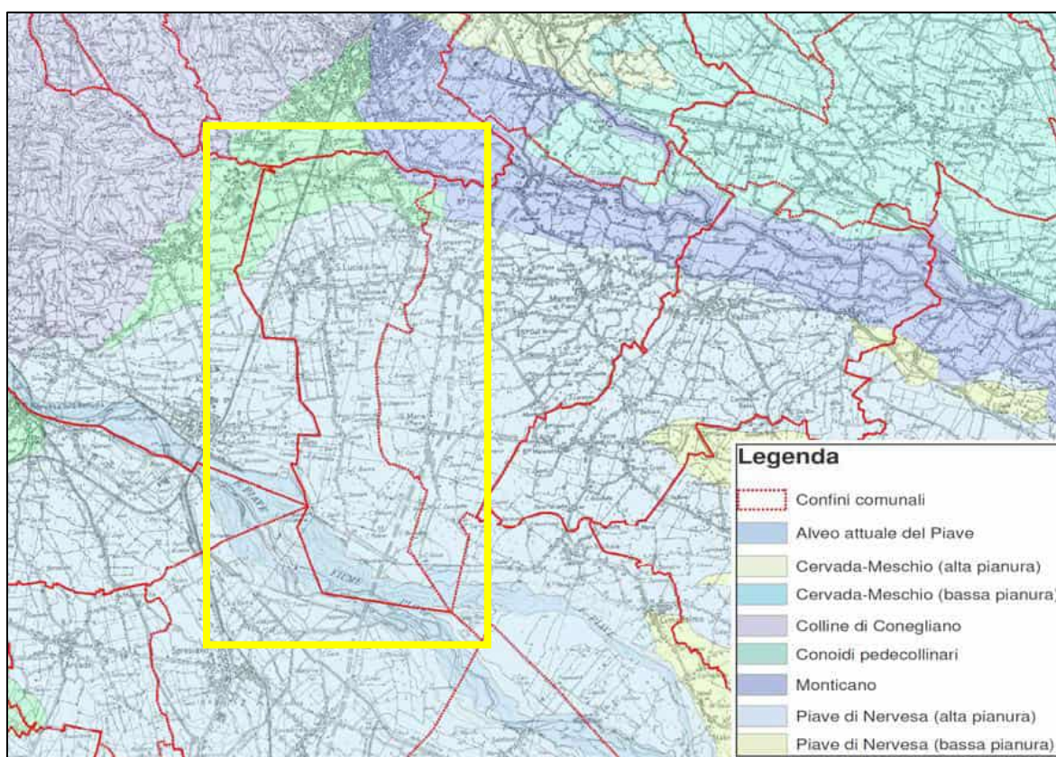
Figura 3. Estratto da Carta geomorfologica della provincia di Treviso e unità di paesaggio del Piano Territoriale di Coordinamento Provinciale (PTCP) della Provincia di Treviso . Il rettangolo giallo racchiude il Comune di Santa Lucia di Piave.
