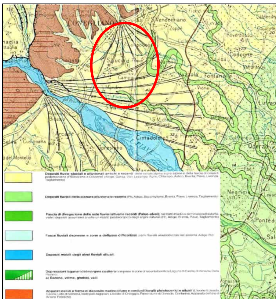
Figura 1. Carta delle Unità Geomorfologiche (Estratto da Regione del Veneto - Carta delle Unità Geomorfologiche alla scala 1:250.000 ).
