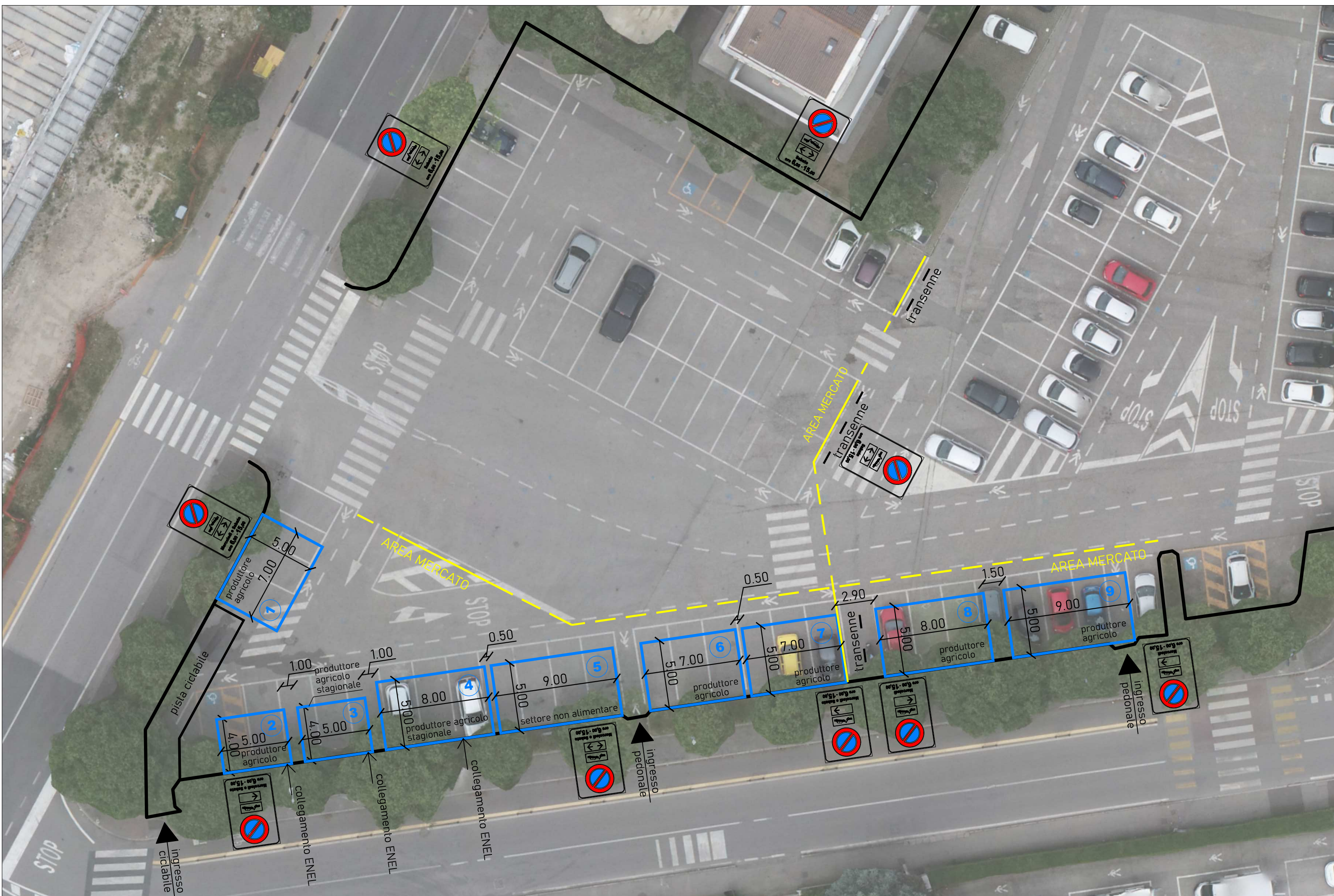
SETTORE VI - Tecnico - Edilizia pubblica - Patrimonio PIAZZALE BACHELET - SISTEMAZIONE MERCATO SETTIMANALE DEL MERCOLEDI'
