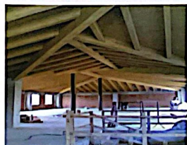
PARTICOLARE DELLA TRAMA LIGNEA DEL TETTO
