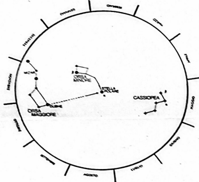
FIG. 1 - Il cielo del nord. Per conoscere la posizione in cielo, alle ore 21, delle principali costellazioni (Cassiopea e le Orse), ruotare la pagina in modo da leggere in basso il nome del mese preso in esame. Tenendo presente che ogni tacca vale 3 ore, per tempi antecedenti le 21 o successivi ruotare rispettivamente in senso orario e antiorario.
