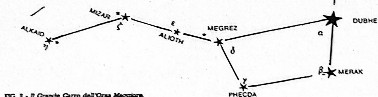
FIG. 2 - Il Grande Carro dell'Orsa Maggiore.
