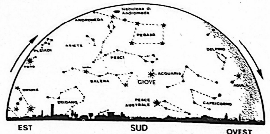
FIG. 3 - Il cielo del sud in autunno alle ore 21 circa.
