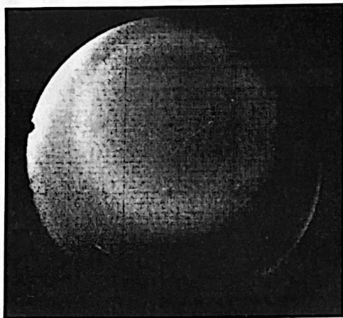
Fig. 1 - Urano in un'immagine inviata dalla sonda Voyager 2, successivamente rielaborata a terra
