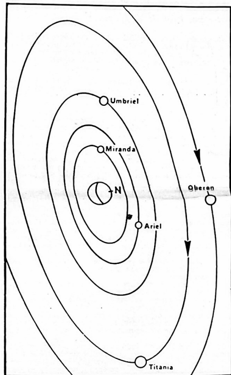
Fig. 4 - I satelliti maggiori di Urano, giacenti nel piano equatoriale (come gli anelli) hanno rivoluzione retrograda, cioè oraria
