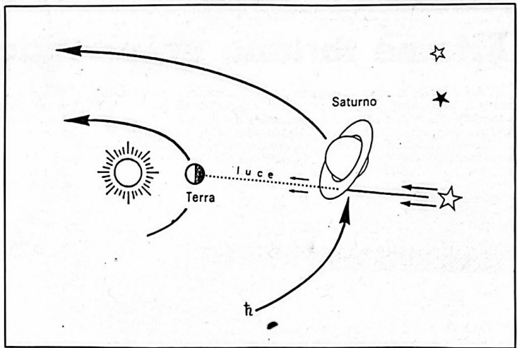
Fig. 1 Per illustrare una delle conferme sperimentali della teoria di Maxwell, secondo cui gli anelli di Saturno non possono essere un corpo solido, ma debbono essere costituiti da una miriade di particelle di varia dimensione. Quando per caso gli anelli di Saturno occultassero una stella (massimamente l'anello A), la luce dall'astro riuscirebbe ad attraversare l'ostacolo e a giungere, sia pure molto ridotta, fino alla Terra. Ciò dimostra ampiamente che gli anelli sono trasparenti, quindi non solidi.
