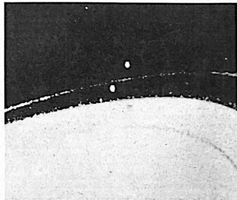
Fig. 3 L'anello F tra i due satelliti pastore prossimi alla congiunzione.
