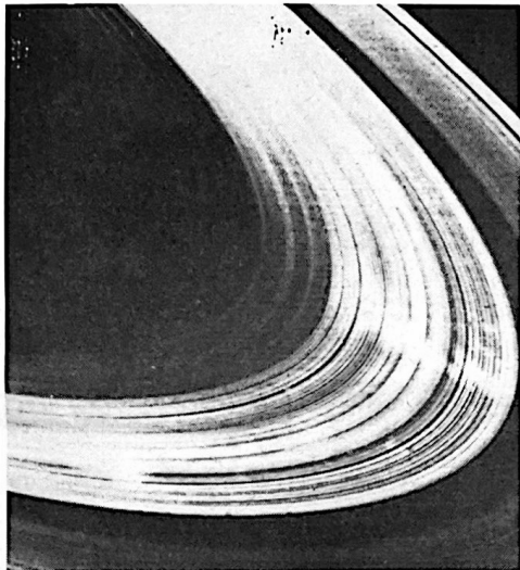
Fig. 2 Gli anelli visti dalla sonda: appaiono come un disco microscopico. L'anello B è il più chiaro e sinistra, l'anello A è quello chiaro a destra. Fra i due in nero la divisione di Cassini.
