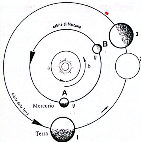
Fig. 1 - Per illustrare il periodo sinodico di Mercurio (intervallo temporale tra due fasi identiche). Mentre Mercurio compie una rivoluzione (periodo siderale, indicato dal cerchio interno "a") in 88 giorni, partendo dalla posizione "A" (congiunzione inferiore, fase di pianeta nuovo) e ritornando in "A", la Terra dalla posizione "1" si porta nella posizione "2", percorrendo circa 1/4 della sua orbita. Mercurio, per ritornare nelle condizioni di partenza rispetto alla Terra ed al Sole, cioè per riproporre ancora la fase nuova (alla congiunzione inferiore), deve portarsi in "B", raggiungendo così la Terra che nel frattempo si è trasferita nella posizione "3". A percorrere l'arco "AB" della propria orbita, Mercurio impiega 23 giorni (tale periodo è indicato internamente dalla posizione di circonferenza "b"). Il periodo sinodico di Mercurio sarà pertanto di (88+23) 116 giorni. In figura tale intervallo temporale è materializzato dalla "a" e da "b": a + b indica infatti il cammino di Mercurio per passare da una fase nuova alla successiva.
