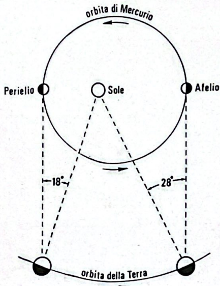
Fig. 2 - Data la forte eccentricità dell'orbita ( e=0,2 ), le elongazioni massime di Mercurio non hanno tutte lo stesso valore. Quindi non sono egualmente favorevoli per l'osservazione. L'elongazione massima della maggiore ampiezza si realizza allorché il pianeta si trova in afelio: è di 28^\circ ; quella di minore ampiezza ( 18^\circ ) capita quando il pianeta è in perielio. Tuttavia neppure la concomitanza di una circostanza favorevole quale un elevato valore dell'angolo fra orizzonte ed eclittica (che si verifica, come è noto, al mattino ad oriente in autunno e alla sera ad occidente in primavera) può evitare a Mercurio, sia pure in elongazione massima afelica, di essere circondato dai raggi solari.
