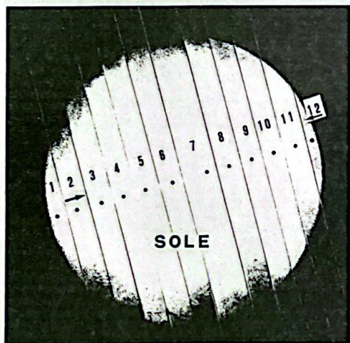
Fig. 3 - Passaggio di Mercurio (che appare come un cerchietto nero) sul disco del Sole. 10 novembre 1973. Ciascuna delle dodici "strisce" numerate (che insieme ricompongono qui il disco solare) è la fotografia di Mercurio e di una porzione di Sole ad un determinato istante. Le ore e i minuti primi (in Tempo Universale o Tempo medio di Greenwich) indicanti il momento del fenomeno (durato in tutto meno di cinque ore) sono, per le singole "strisce": n. 1 = 8h 15'; n. 2 = 8h 40'; n. 3 = 9h 5'; n. 4 = 9h 30'; n. 5 = 9h 55'; n. 6 = 10h 33'; n. 7 = 11h 15'; n. 8 = 11h 40'; n. 9 = 12h 5'; n. 10 = 12h 30'; n. 11 = 12h 55'; n. 12 = 13h 13'. Successivamente vi è stato un solo altro transito, quello del 13 novembre 1986; il prossimo sarà il 6 novembre 1993.
