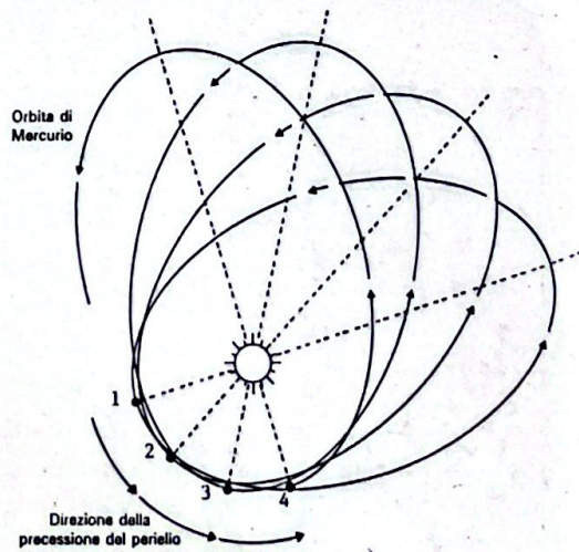
Fig. 5 - Spostamento o avanzamento o precessione del perielio.
