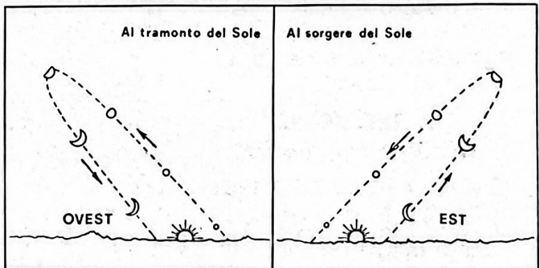
Fig. 4 - Quando è stella della sera, il pianeta interno si avvicina alla Terra; perciò la sua luminosità va aumentando. Quando è stella del mattino si allontana.
