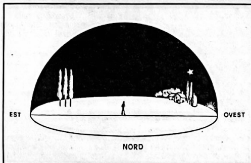
Fig. 2 - Venere, quando segue il Sole, cioè si trova alla sua sinistra, ad Est di esso (elongazione Est) si presenta come stella della sera.
