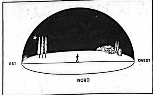
Fig. 3 - Venere, come stella del mattino: precede il Sole trovandosi alla sua destra, cioè ad Ovest di esso (elongazione Ovest).
