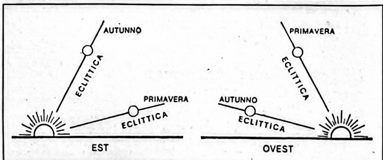
Fig. 5 - L'angolo dell'orizzonte con l'eclittica, è grande al mattino in autunno e alla sera in primavera, onde il pianeta interno come astro del mattino apparirà meglio in autunno e come astro della sera in primavera.
