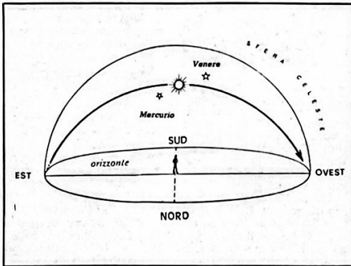
Fig. 1 - I pianeti interni accompagnano il Sole nel suo moto diurno apparente e pertanto si trovano nel cielo del Sud in pieno di. Perciò ad occhio nudo risultano invisibili perché "cancellati" dalla luce solare.
