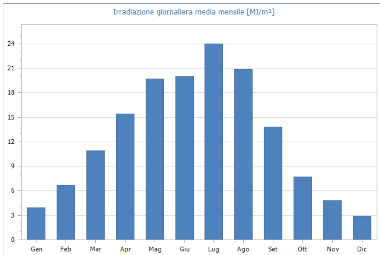
Fig. 1: Irradiazione giornaliera media mensile sul piano orizzontale [MJ/m 2 ]- Fonte dati: UNI 10349:2016 - Stazione di rilevazione: Cinisello Balsamo
