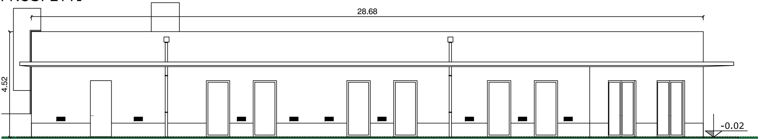
PROSPETTO SUD
