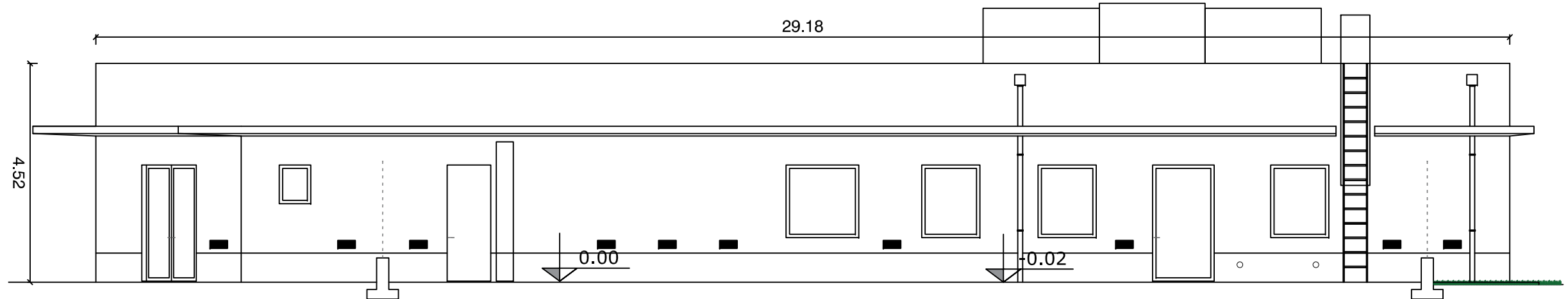
PROSPETTO OVEST
