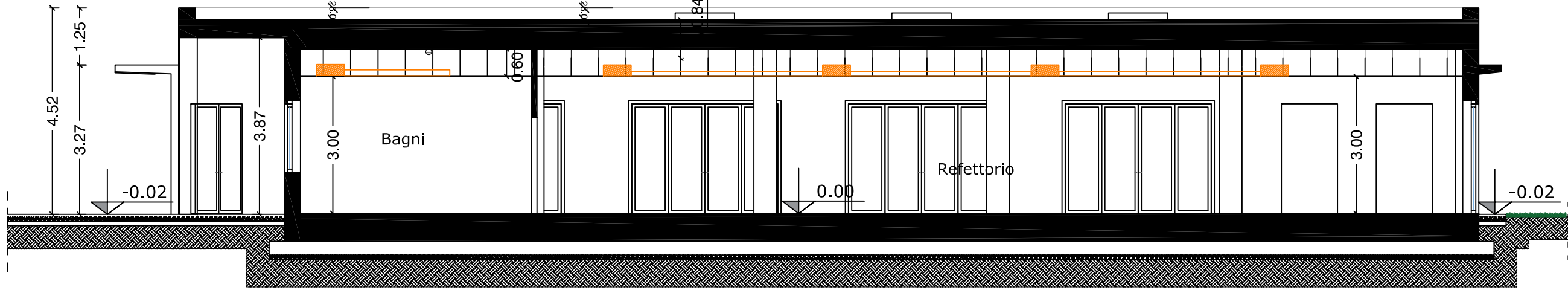
SEZIONE B-B
