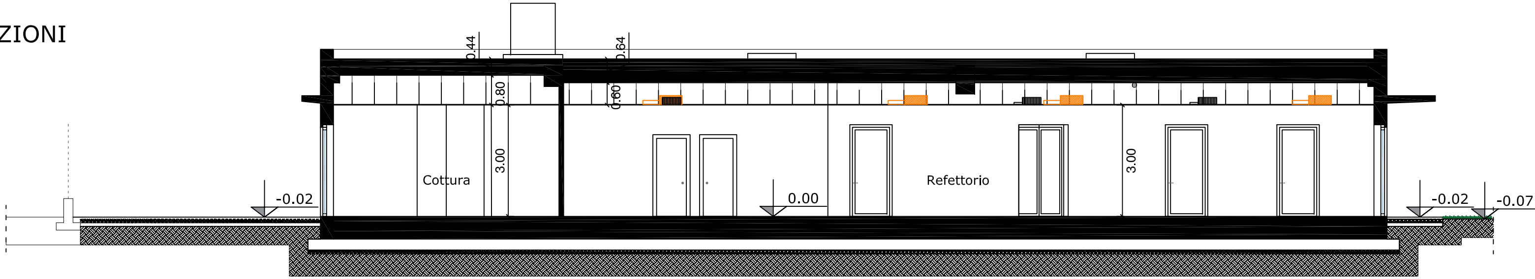
SEZIONE A-A
