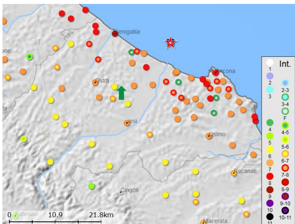
Fig. 21) Terremoti del Catalogo Parametrico dei Terremoti Italiani (CPTI 15 v4.0) dall'anno 1000 al 2020: terremoto del 1930 nel senigalliese
