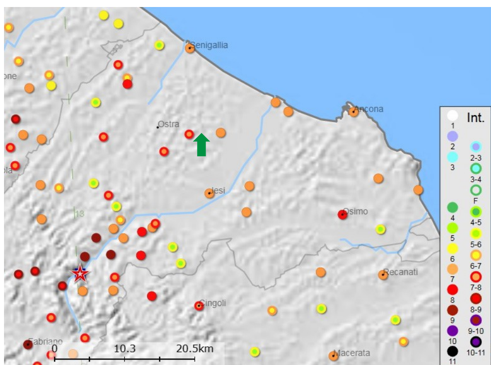
Fig. 20) Terremoti del Catalogo Parametrico dei Terremoti Italiani (CPTI 15 v4.0) dall'anno 1000 al 2020: terremoto del 1741 nel fabrianese
