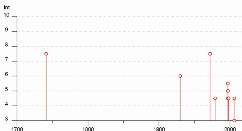
Fig. 18) Grafico INGV - terremoti storici su scala MCS
