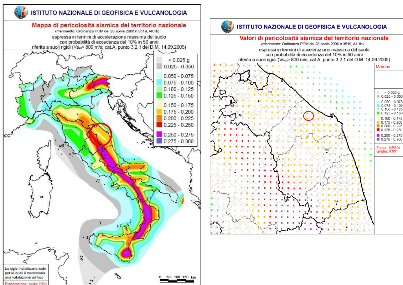
Fig. 16) Mappa di pericolosità sismica del territorio nazionale e regionale (nel cerchio si trova il Comune di Morro d'Alba)
