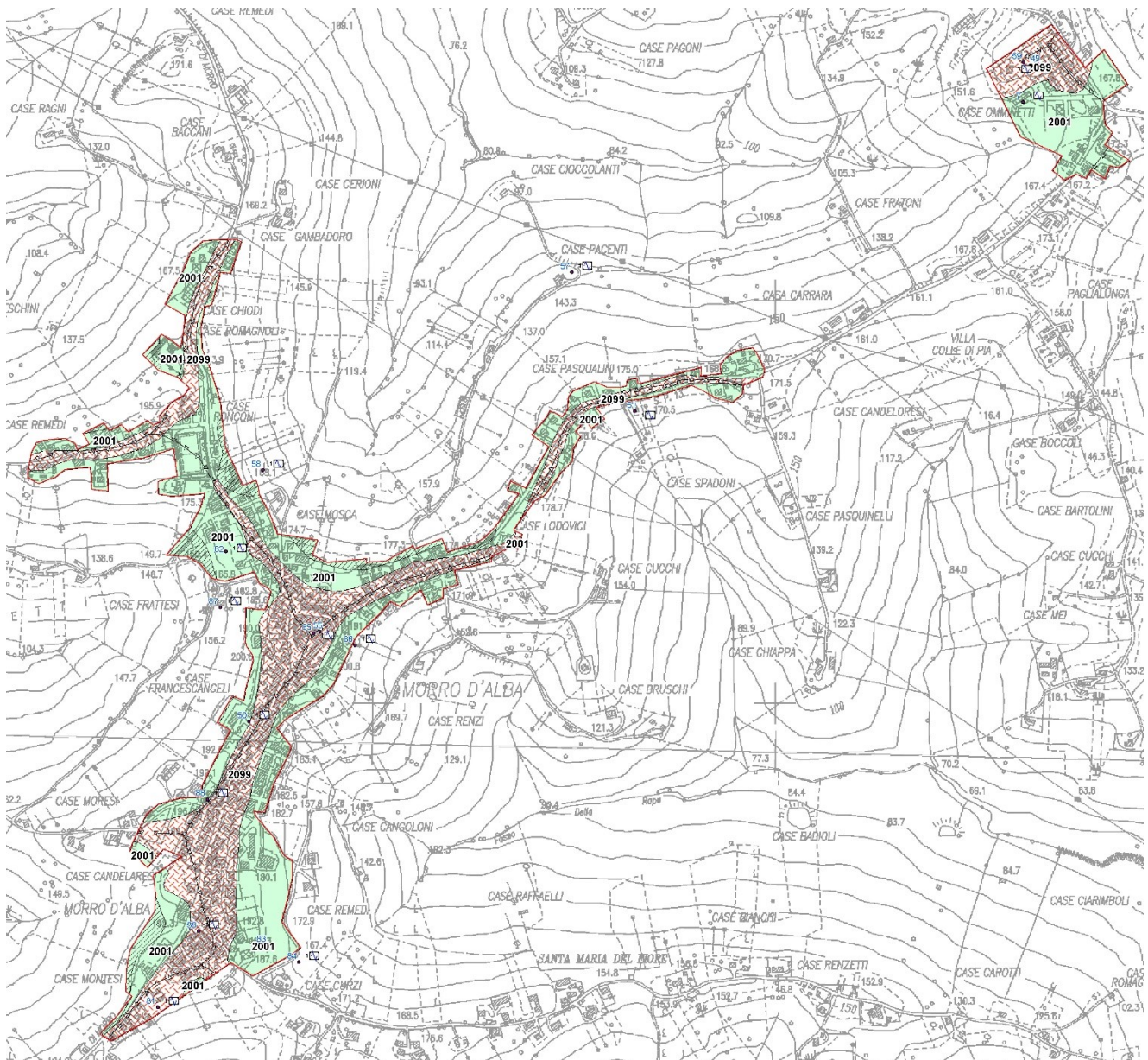
Fig. 22) Stralcio Carta delle MOPS dalla MS 2° livello
