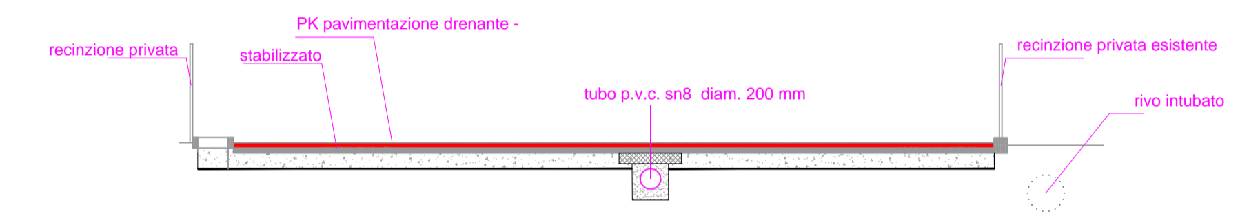
sezione profilo z - z
