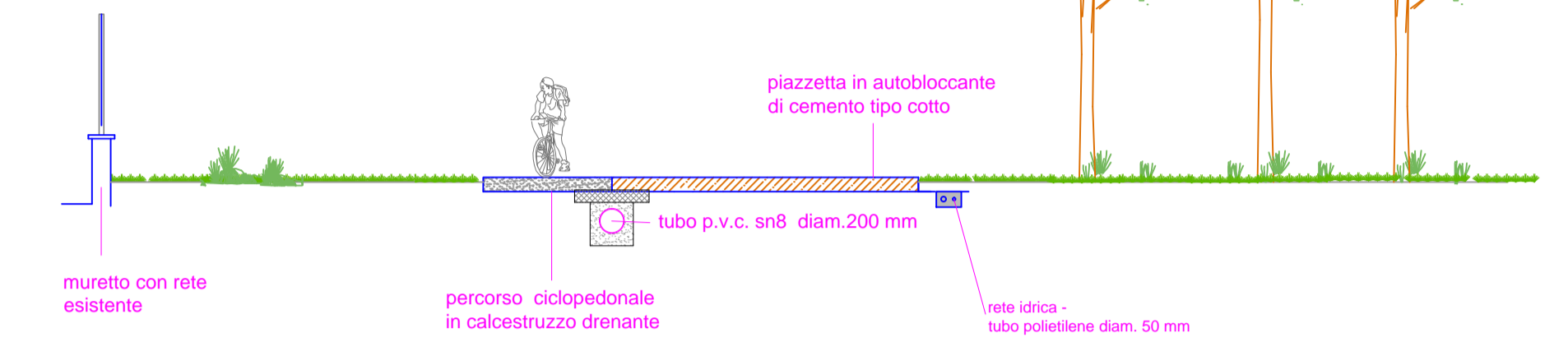
sezione profilo x - x
