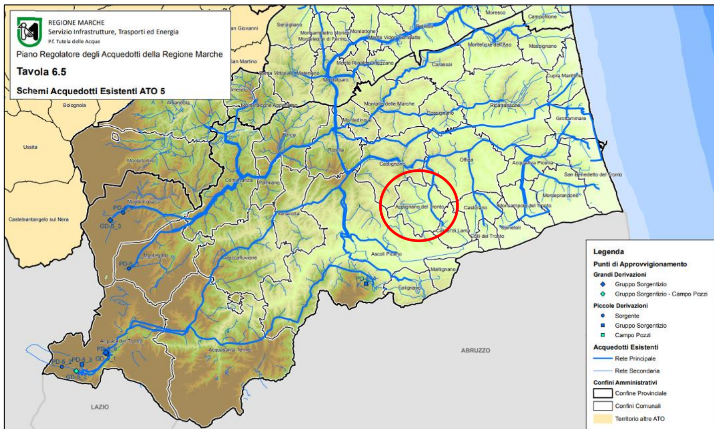
Fig.7: schema acquedotti esistenti – Provincia di Ascoli Piceno
