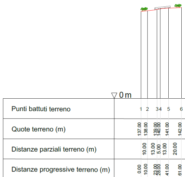
Figura 4 - Sezione AA'
