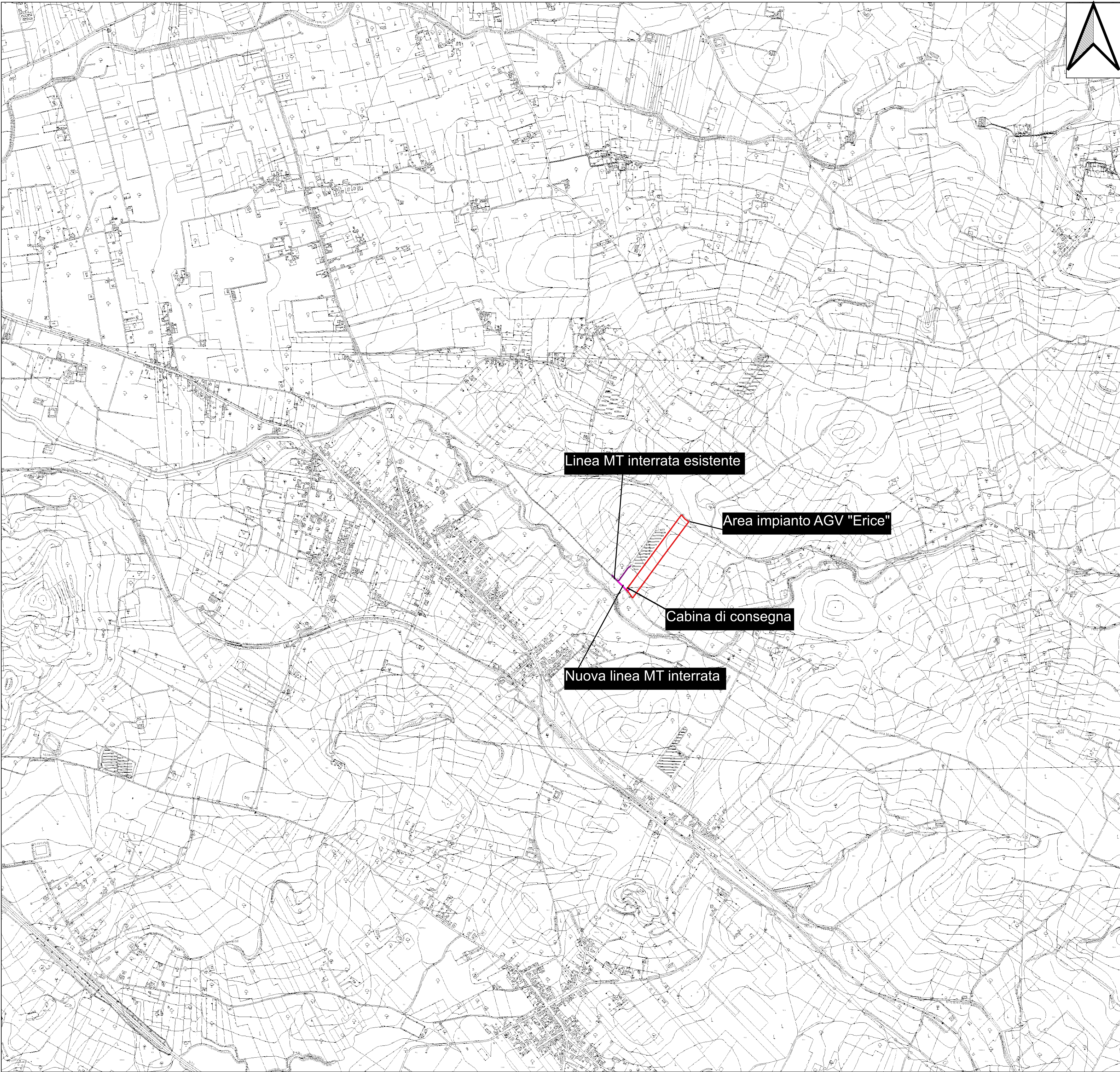
Stralcio "P.A.I." carta del rischio geomorfologico su C.T.R. n.605040. Scala 1:10.000
