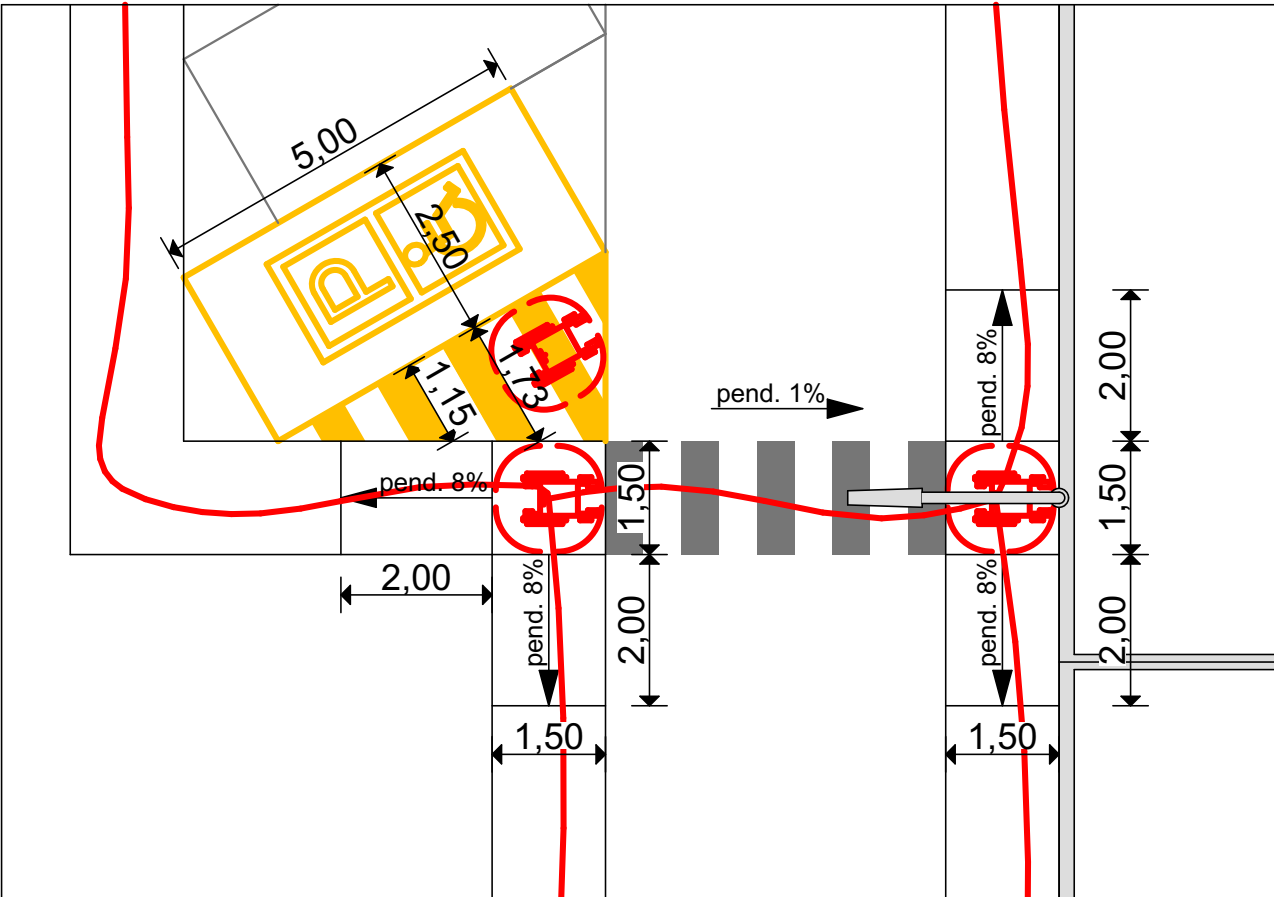
PARTICOLARE n. 7
