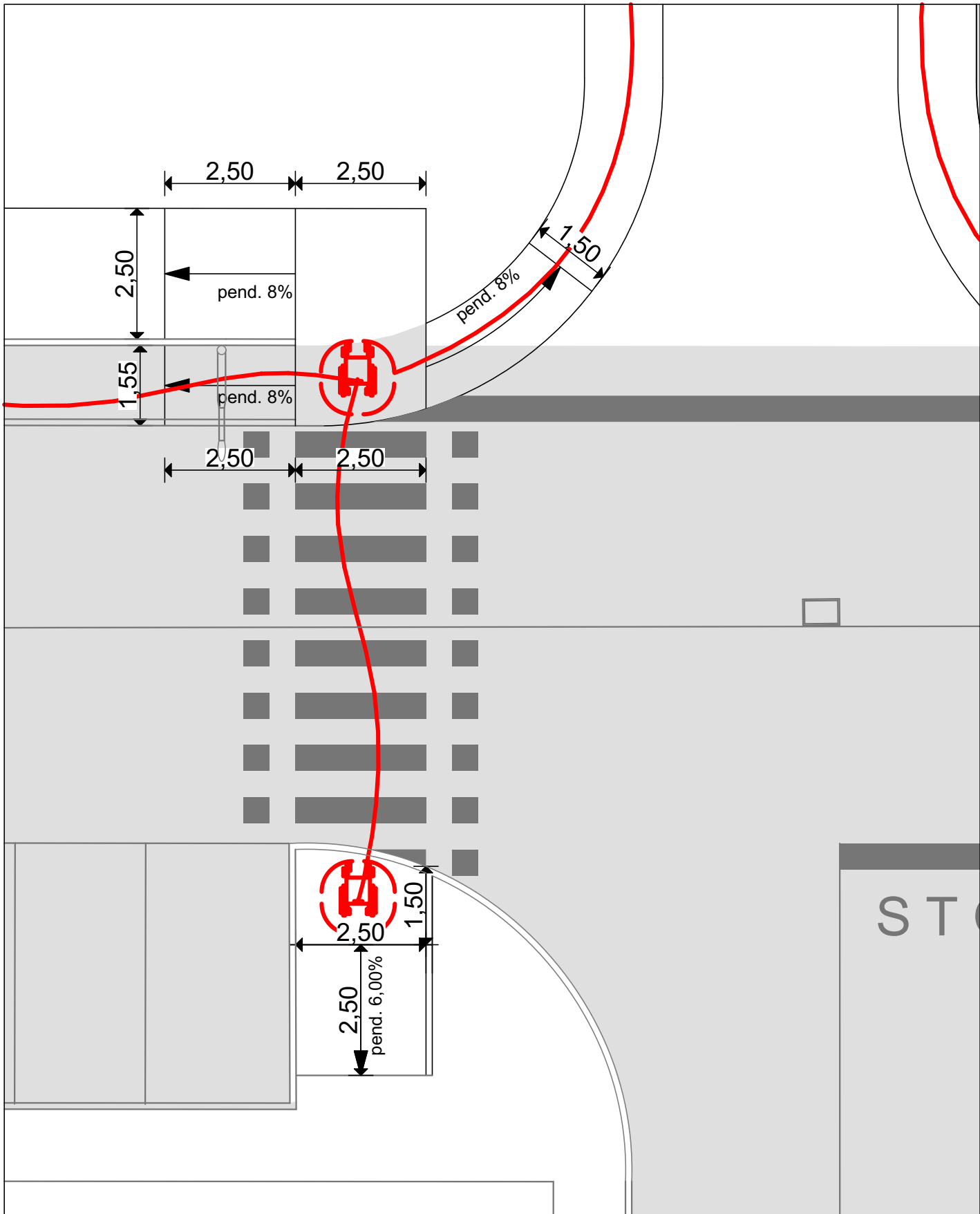
PARTICOLARE n. 9
