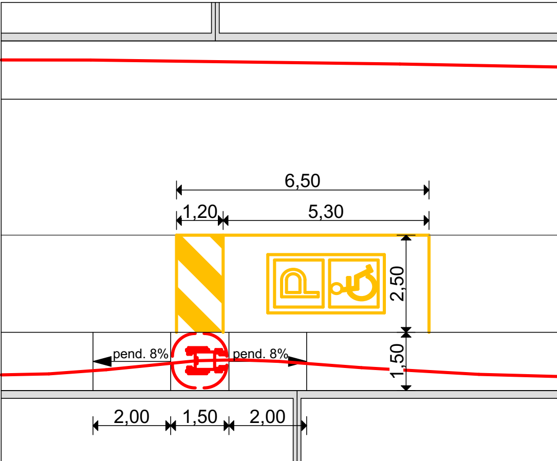
PARTICOLARE n. 6
