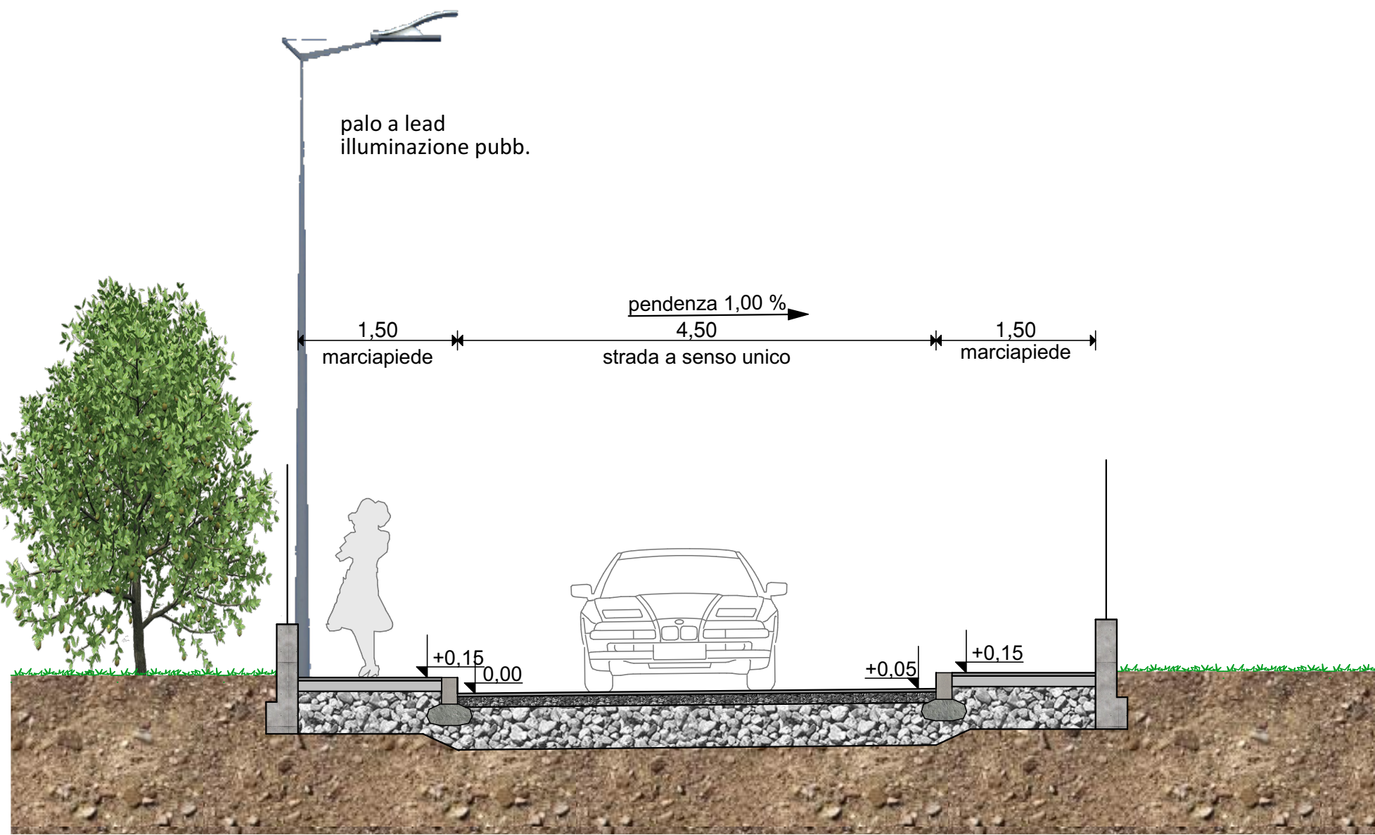
SEZIONE TIPO 4-4
