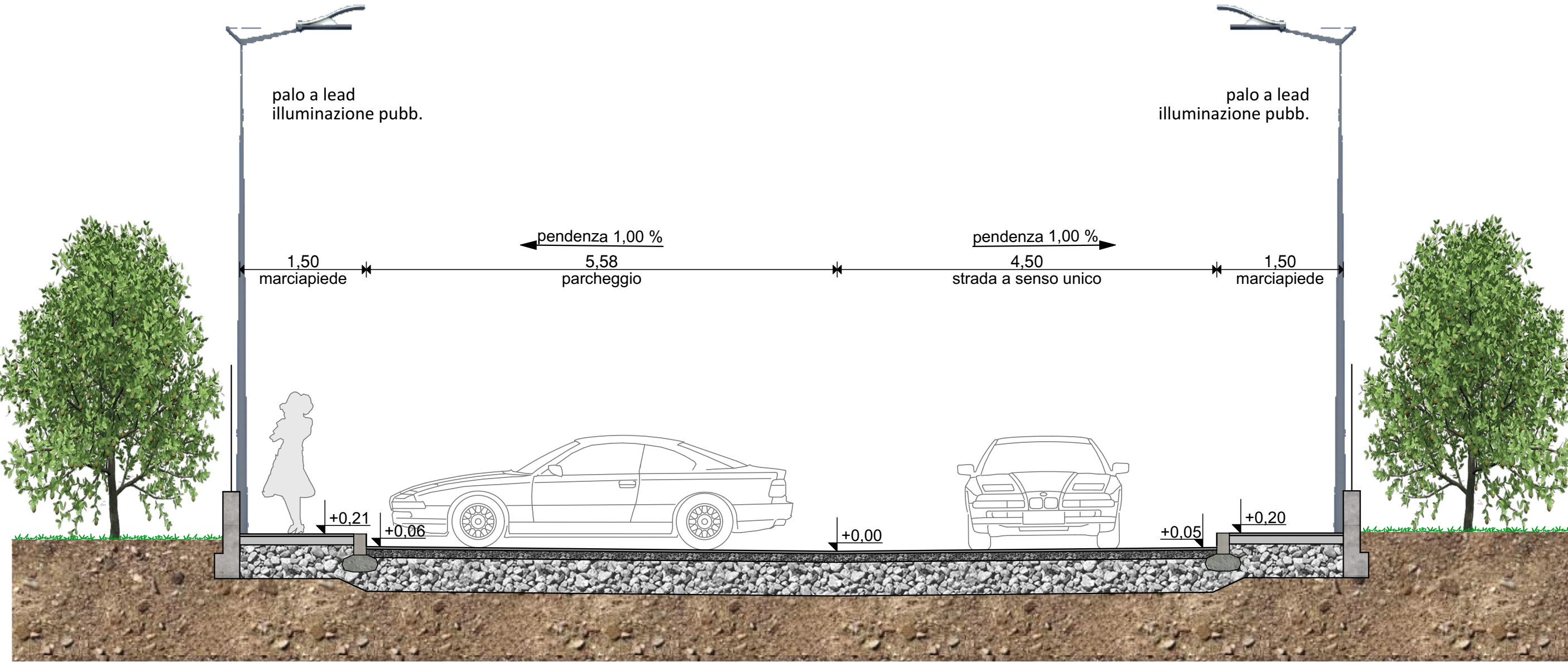
SEZIONE TIPO 3-3
