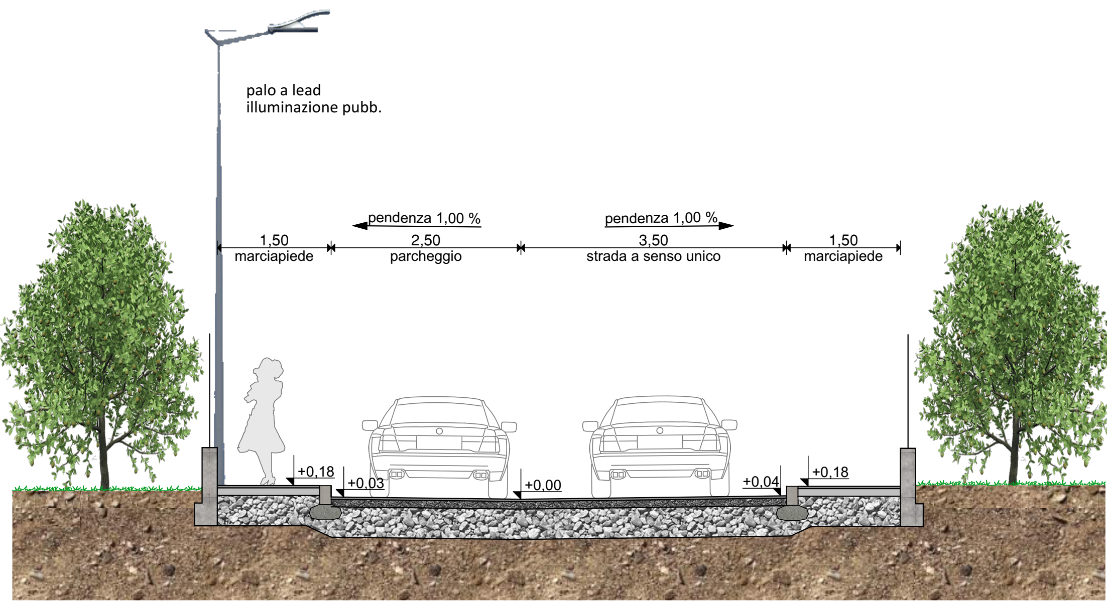
SEZIONE TIPO 2-2
