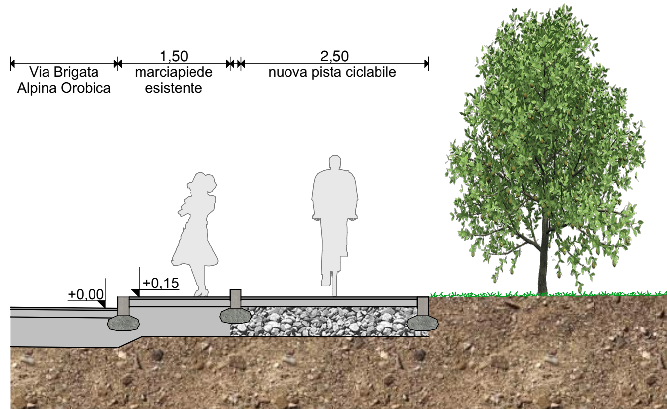
SEZIONE TIPO 5-5
