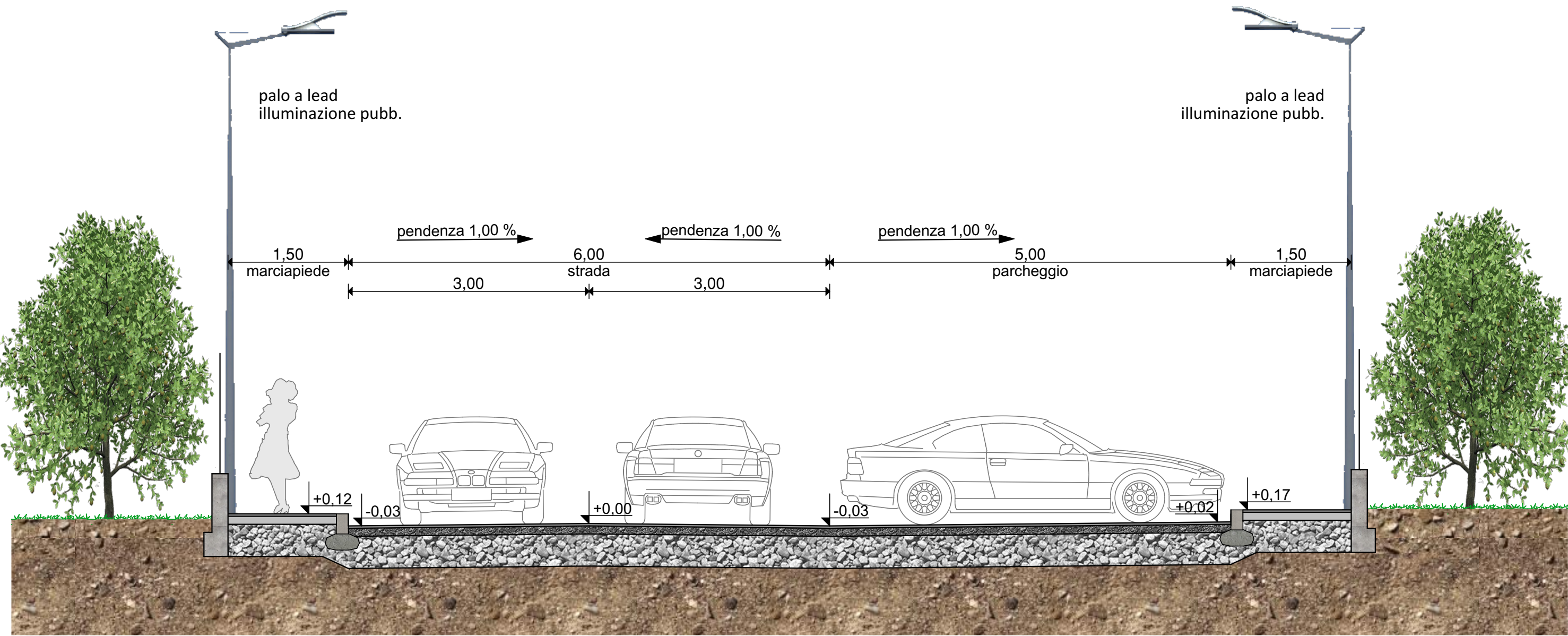
SEZIONE TIPO 1-1
