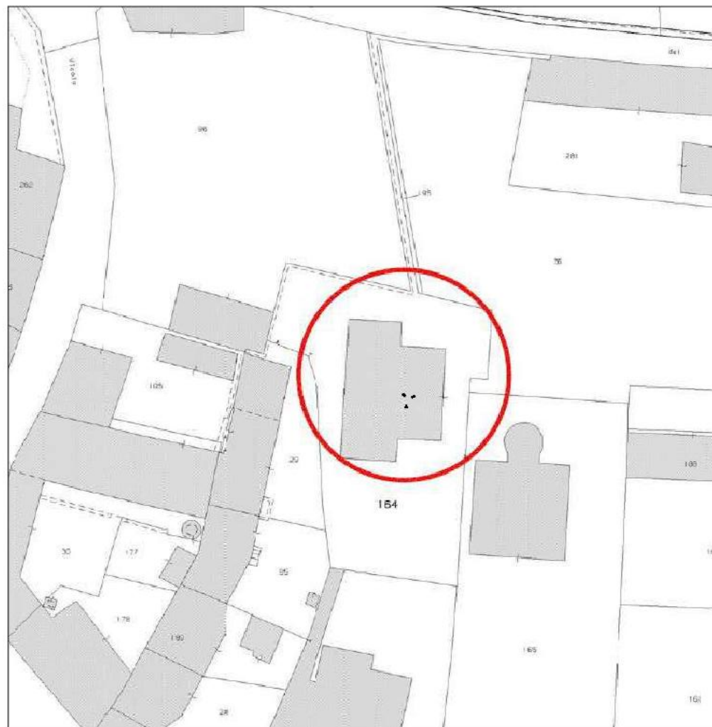
ESTRATTO CATASTALE fg.40 – mapp.164 scala 1:500
