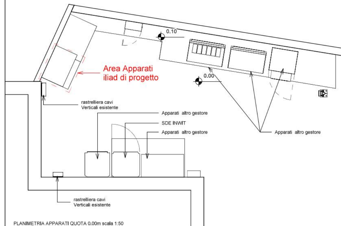
PLANIMETRIA APPARATI QUOTA 0.00m scala 1:50
