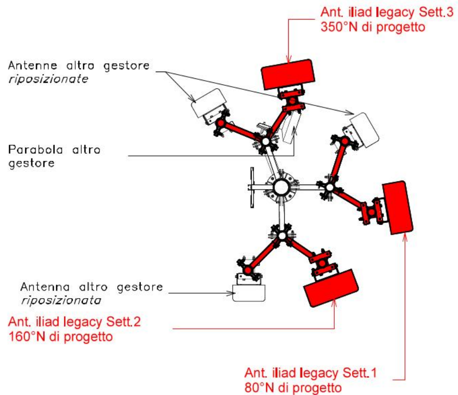
PARTICOLARE ANTENNE QUOTA +15.93m scala 1:25
