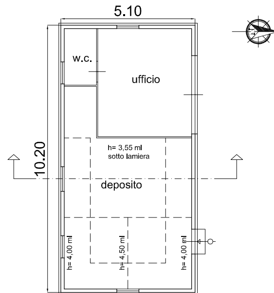
Pianta
