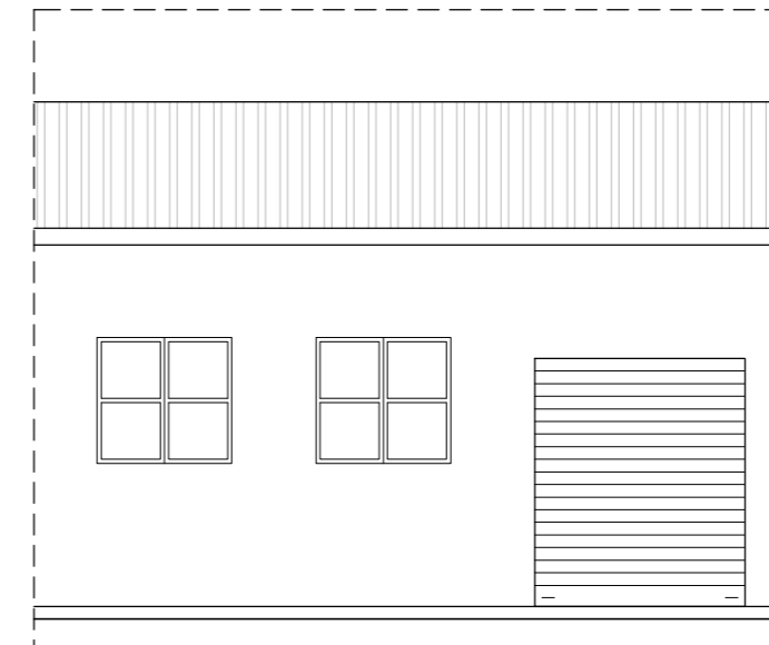
PROSPETTO OVEST
