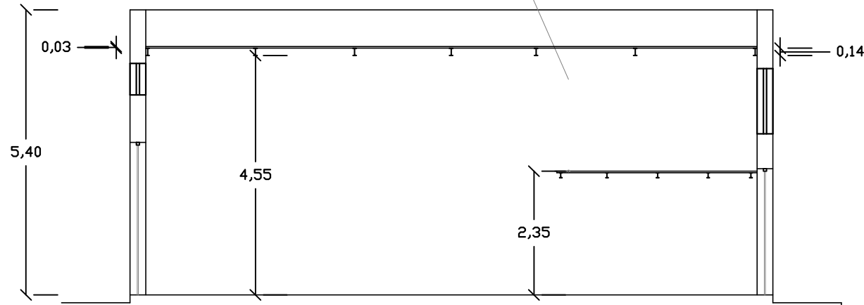
SEZIONE A-A'
