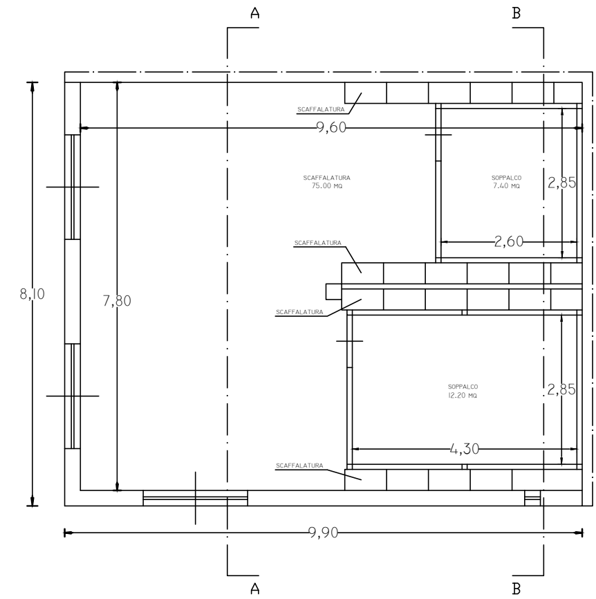
PIANTA PIANO SOPPALCATO
