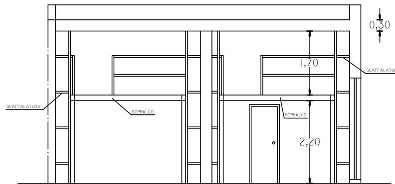
SEZIONE A-A
