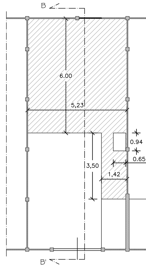
PIANTA PIANO SCAFFALATURA SOPPALCATA
