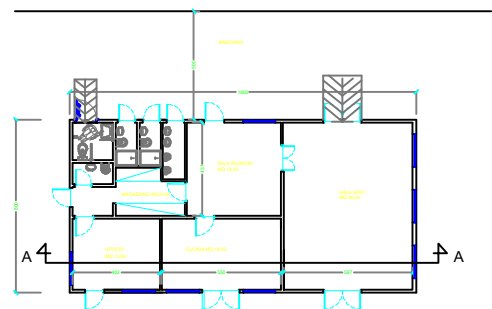
PIANTA PIANO TERRA RAPP. 1:100
