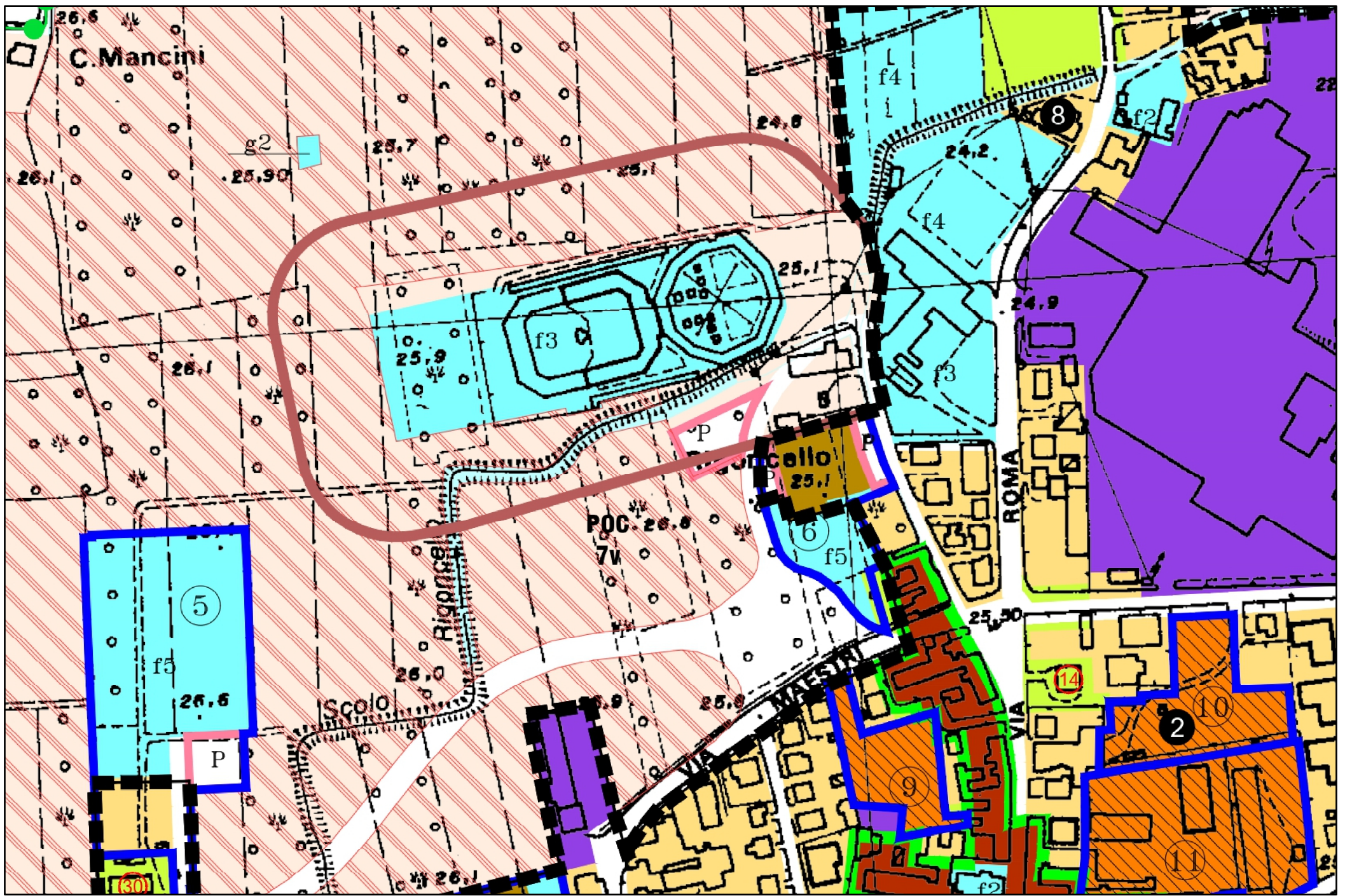
Stralcio della Tav. 1 del RUE - Intero Territorio - STATO VIGENTE in scala 1:2.500
