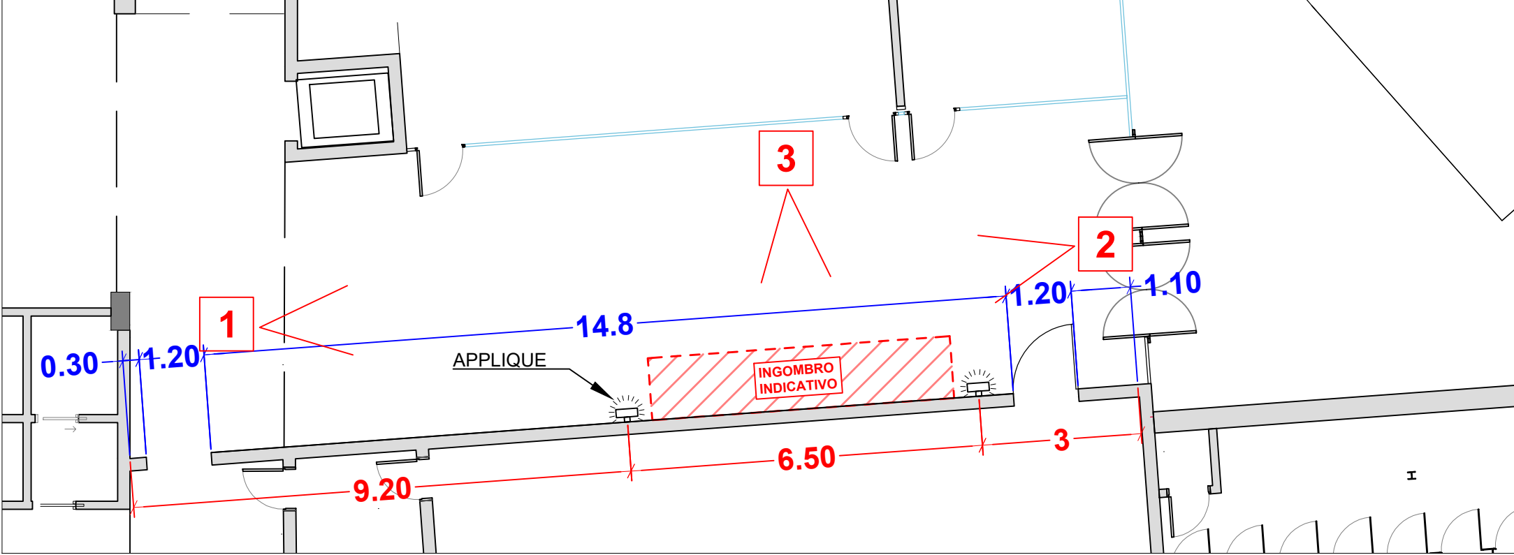
PLANIMETRIA DI DETAGLIO
