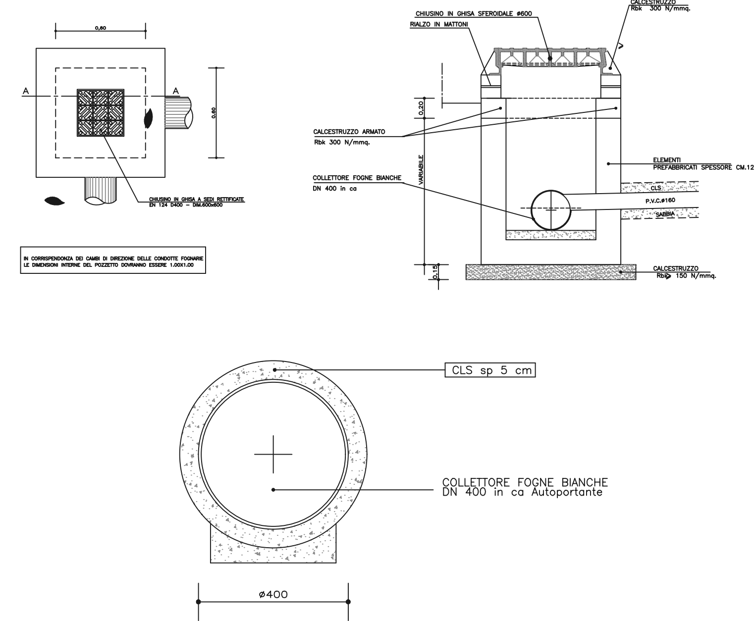
PARTICOLARE POZZETTO D'ISPEZIONE FOGNATURA ACQUE BIANCHE scala. 1:25
