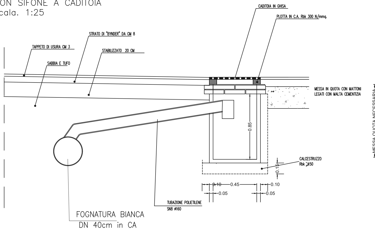
PARTICOLARE POZZETTO CON SIFONE A CADITOIA scala. 1:25
