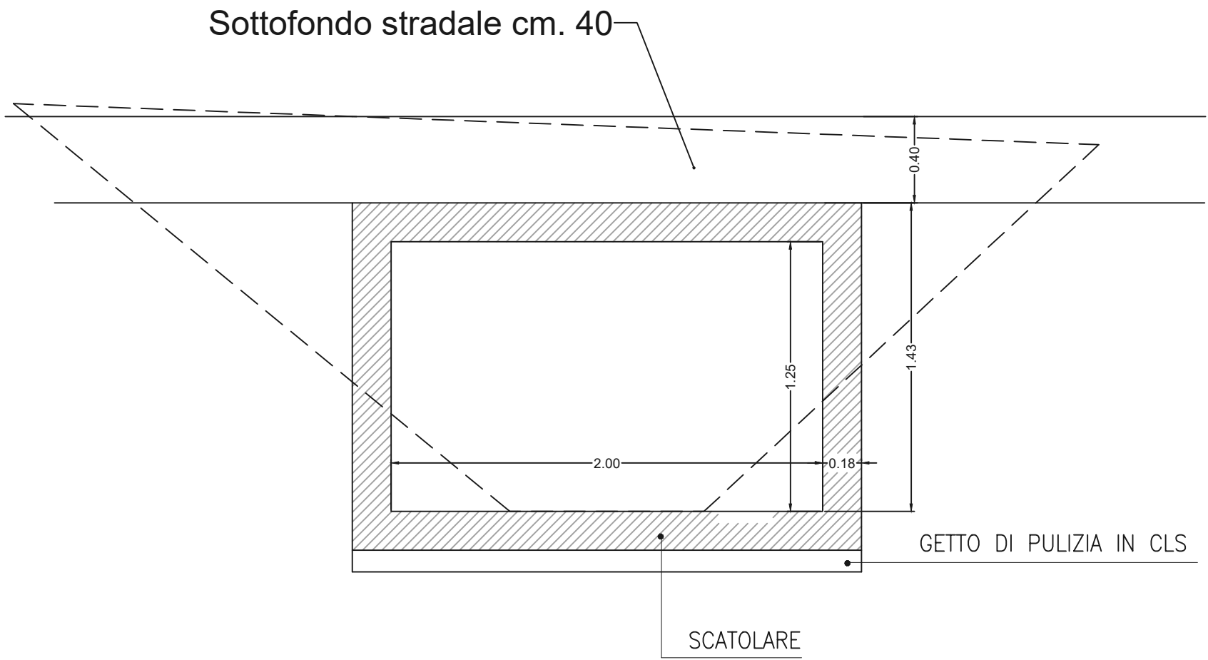
PARTICOLARE SCATOLARE A SEZIONE RETTANGOLARE, PER FOSSE scala. 1:25
