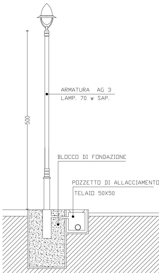
PALO PER ILLUMINAZIONE CICLABILE SCALA 1:50
