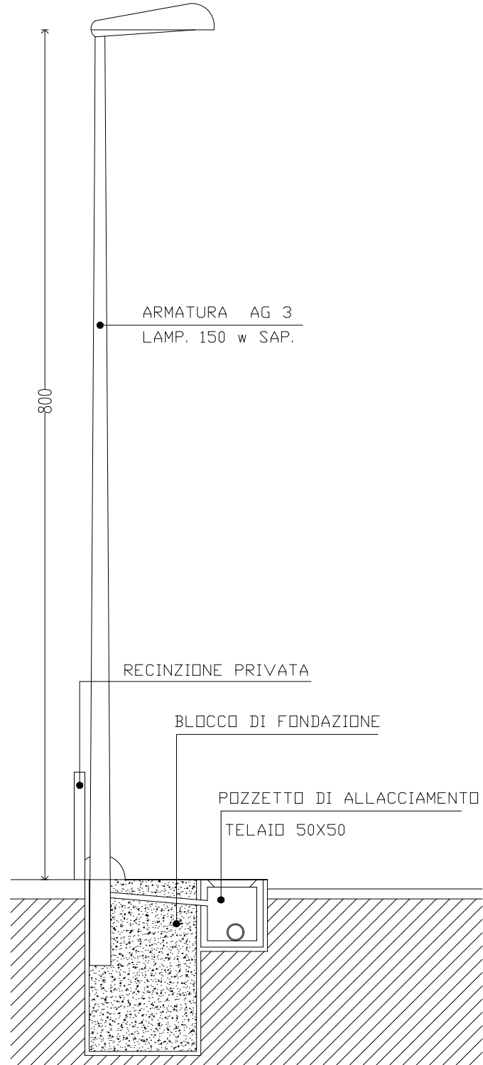
PALO PER ILLUMINAZIONE STRADA SCALA 1:50
