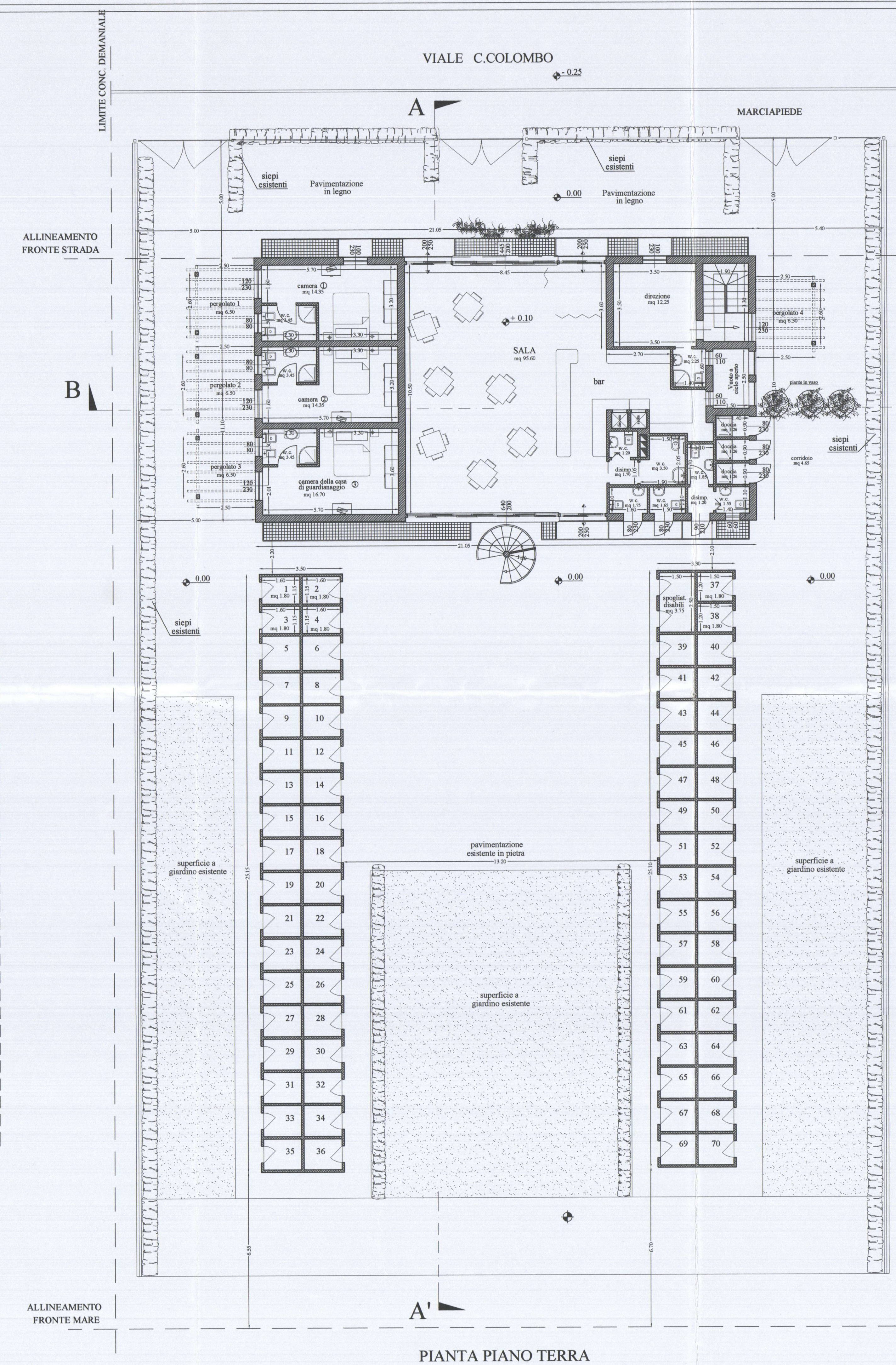
PIANTA PIANO TERRA
