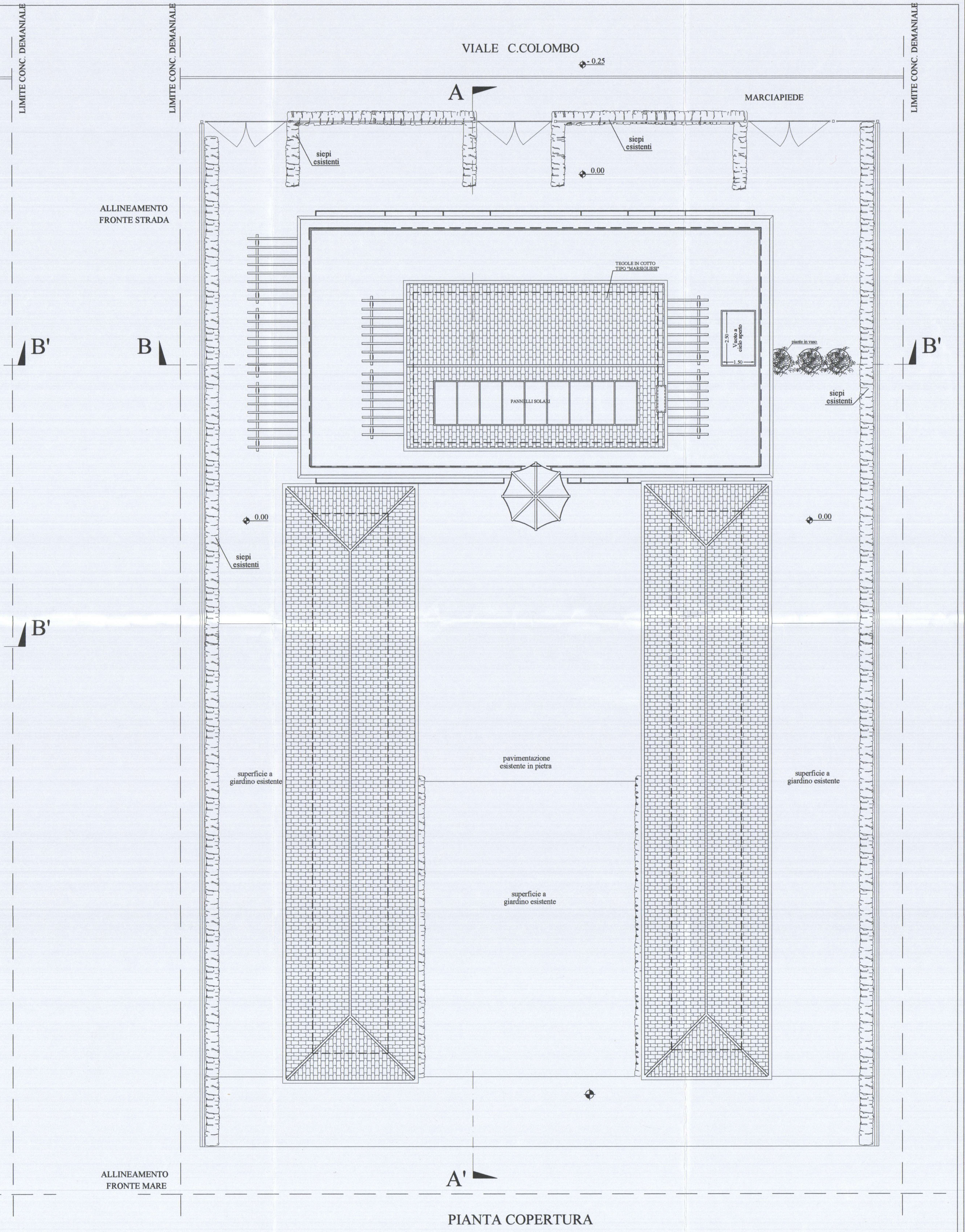
PIANTA COPERTURA
