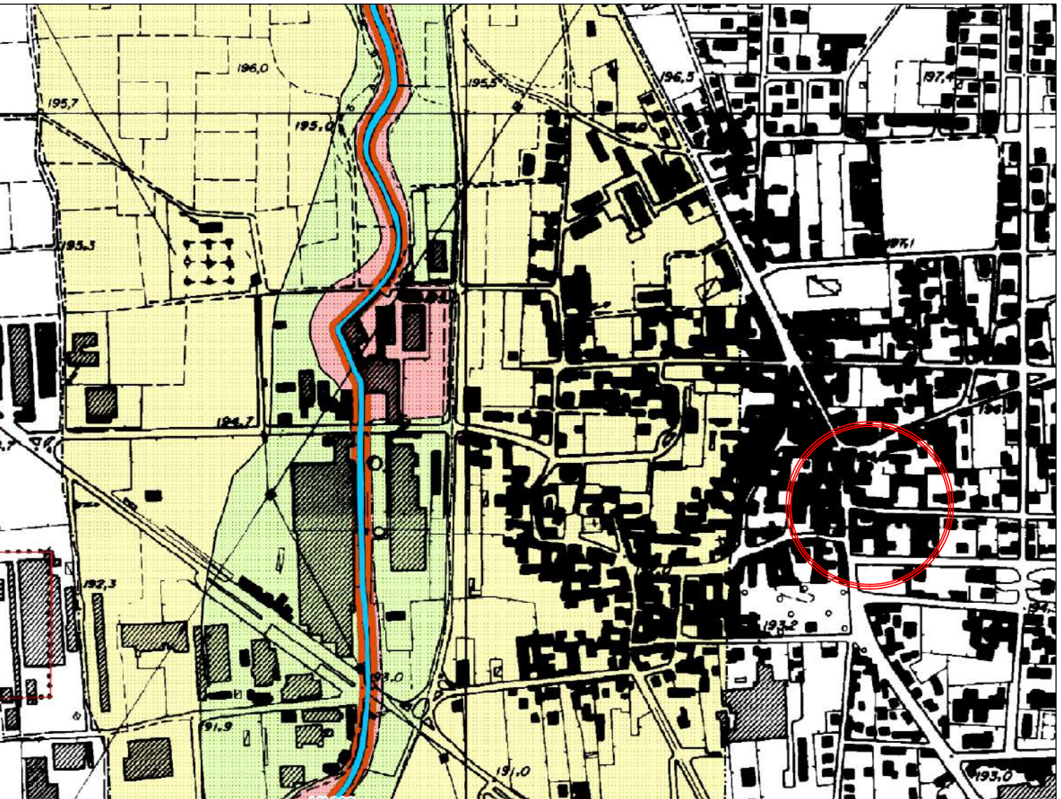
Individuazione del reticolo idrico minore e delle fasce di rispetto - scala 1:5000
