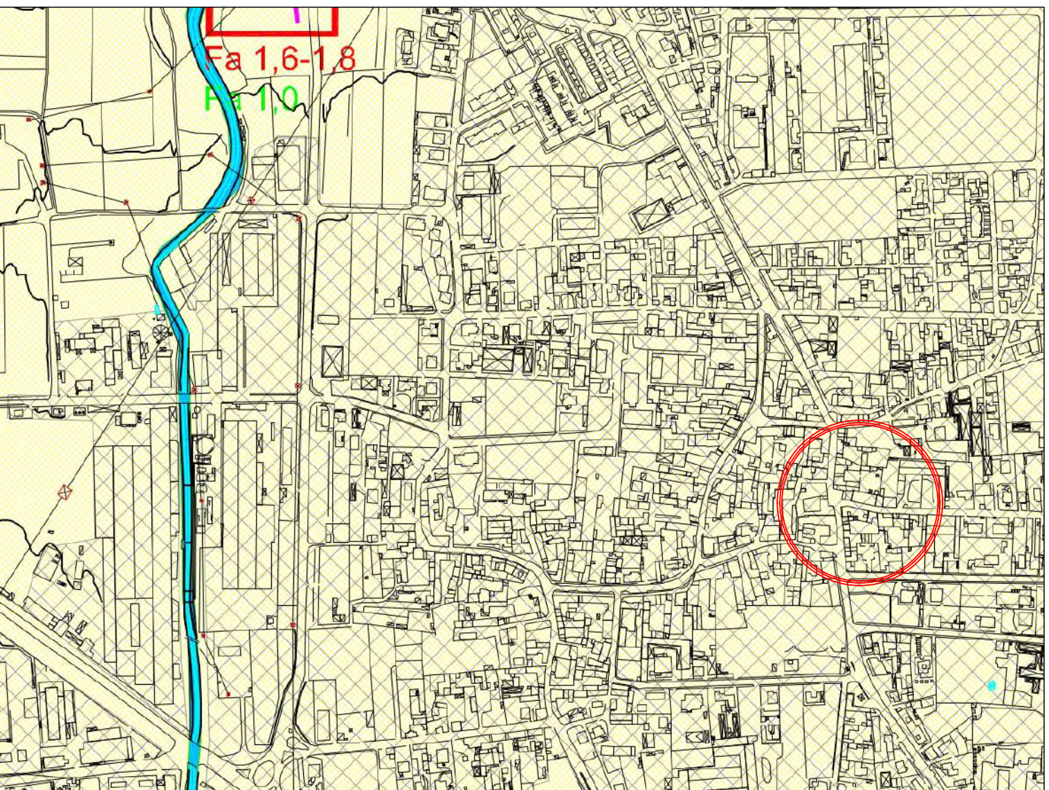
Carta della pericolosità sismica locale - scala 1:5000
