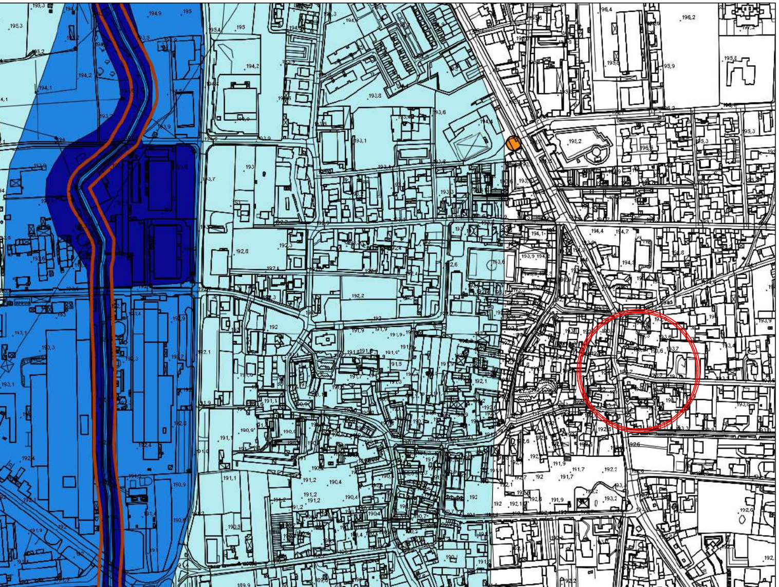
Aggiornamento della componente geologica, idrogeologica e sismica Carta dei Vincoli - scala 1:5000
