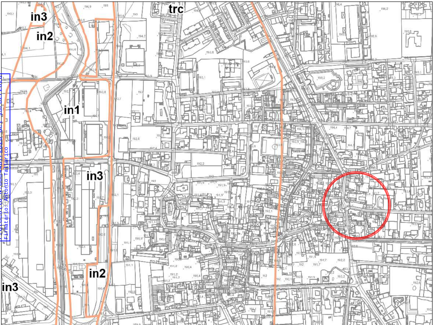
Aggiornamento della componente geologica, idrogeologica e sismica Carta di Sintesi - scala 1:5000
