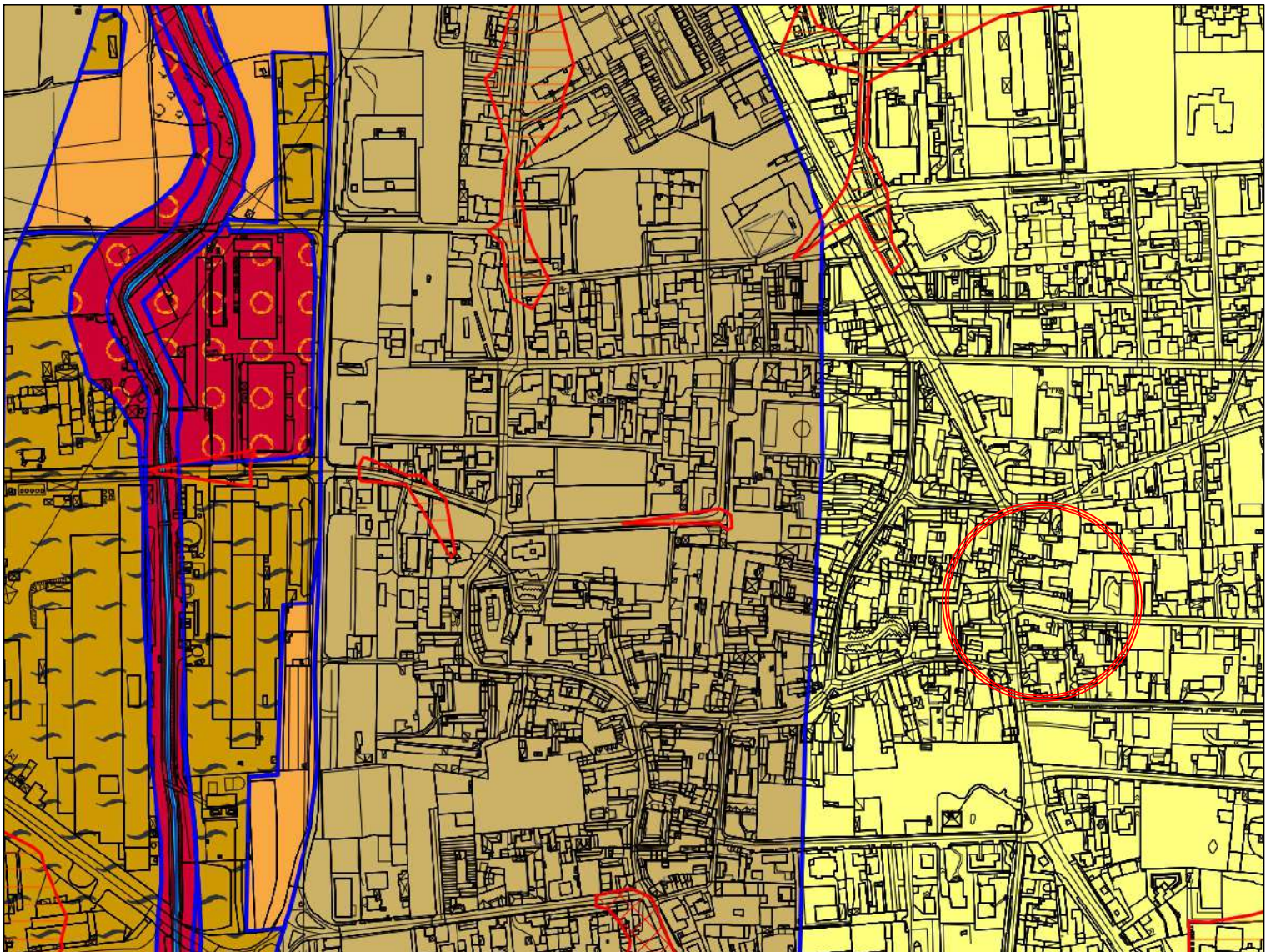
Aggiornamento della componente geologica, idrogeologica e sismica Carta della Fattibilità Geologica - scala 1:5000
