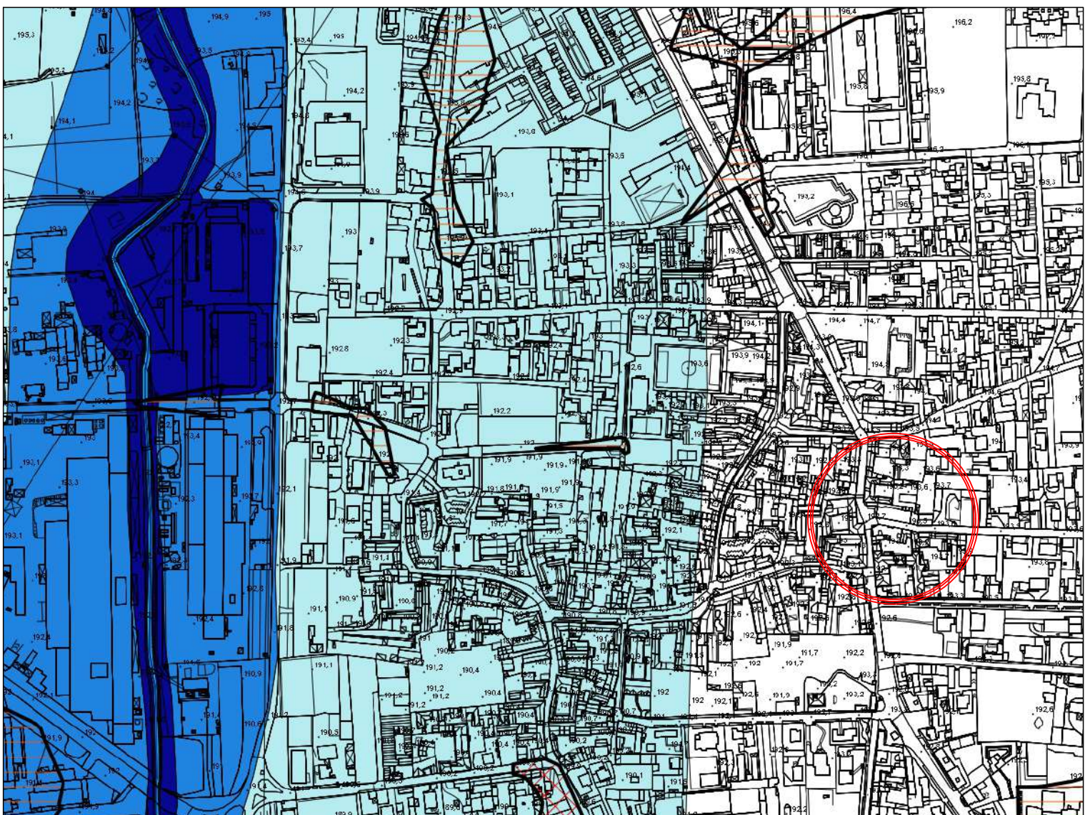
Carta del Rischio Idraulico - scala 1:5000
