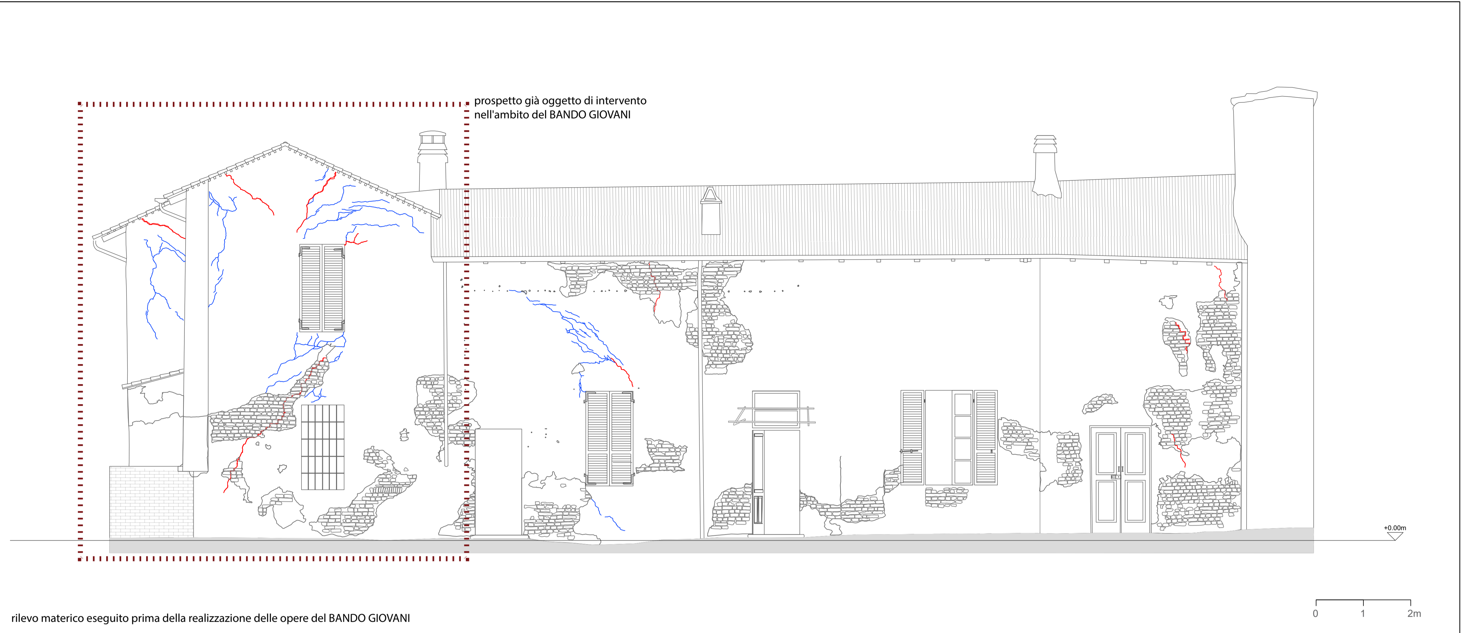
PROSPETTO SUD - OVEST
